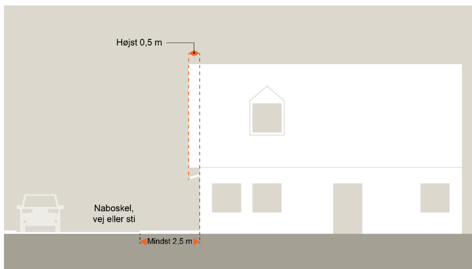
Tegning 24: Afstand til skel ved tagudhæng.
