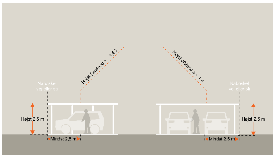
Tegning 14: Højder og afstande for carporte og tilsvarende i skel og skelbremme.
