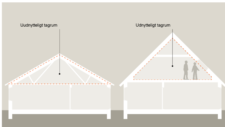
Tegning 19: Udnyttelige og udnyttelige tagrum.
