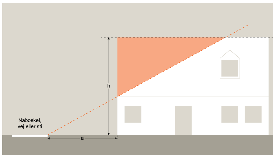
Tegning 21: Gavltrekanth ved taghældning på 45 grader set ved længdefacade.
