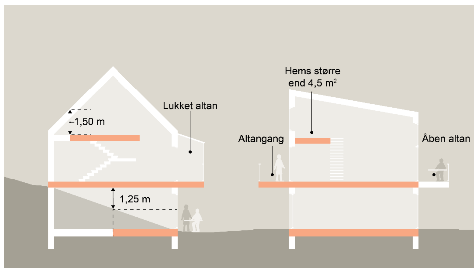
Tegning 2: Figuren til venstre viser det samlede etageareal og figuren til højre viser arealet minus fradrag. Det skal understreges, at en altan,
