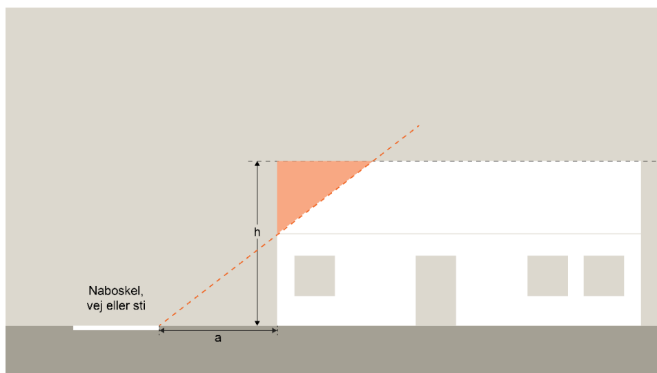
Tegning 23: Gavltrekan ved mindre end 45 graders taghældning set langs længdefacade.
