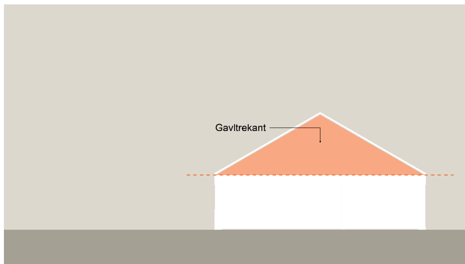
Tegning 22: Gavltrekanth ved mindre end 45 graders taghældning set ved gavlfacade.
