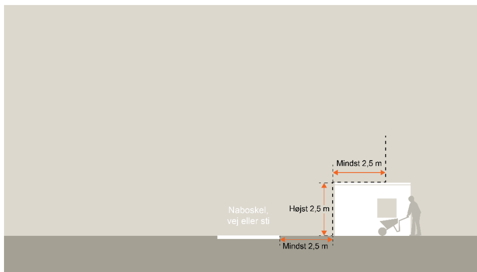
Tegning 15: Højder ved småhuse i skel ved sommerhuse.
