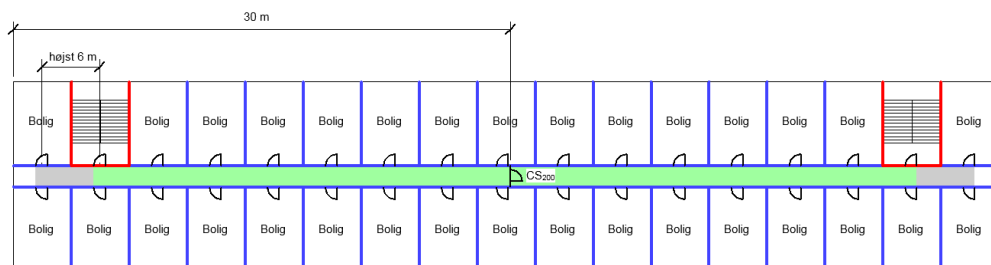
Figur 44 - illustration af referencebyggeriet, grøn farve angiver flugtvejsgang med mulighed for at flygte i to retninger, grå farve angiver områder med mulighed for at flygte i en retning.
