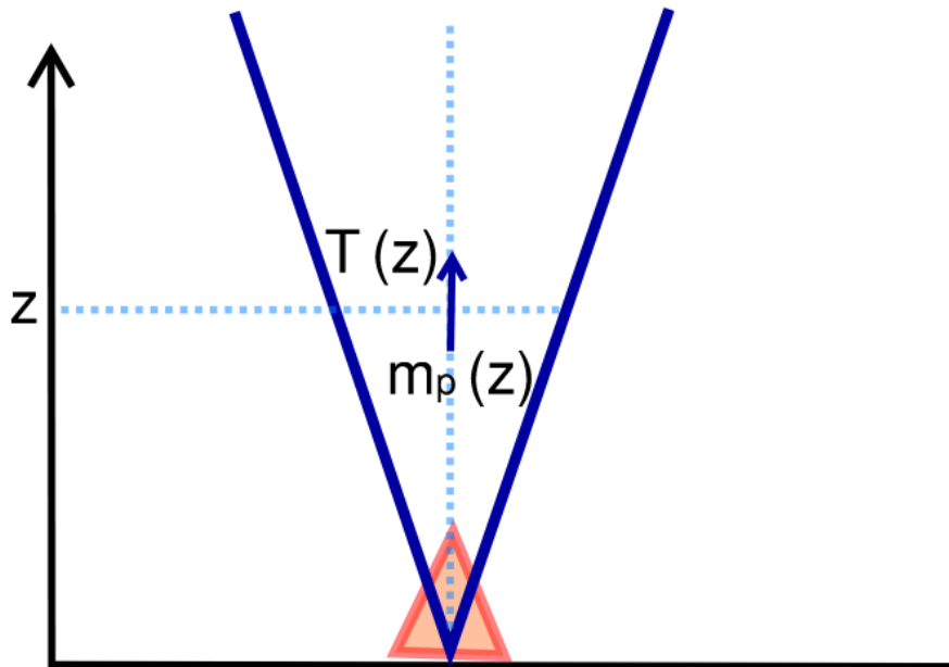
Figur 29: Zukoskis røgfaner
