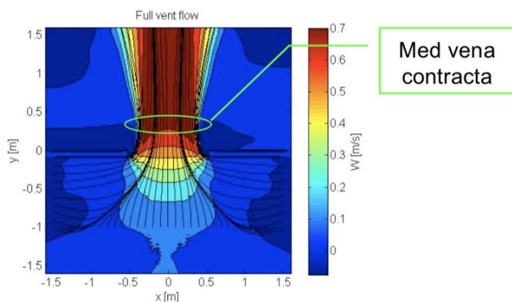
Figur 17: Modelling af blænde for strømning gennem naturlig ventilationsåbning. Lånt fra CFD Best Practice.
