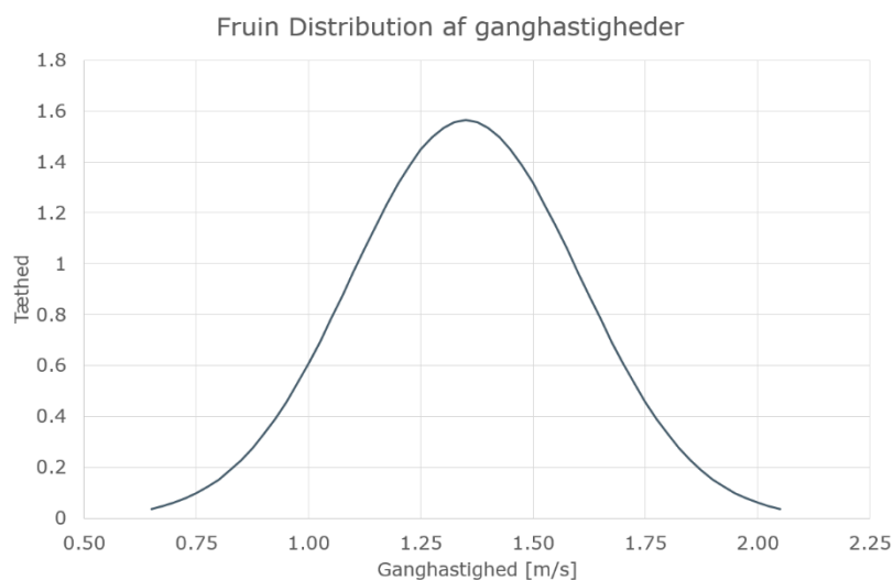
Figur 25: Fordelingen af ganghastigheder i 'Fruin distribution' [19].
