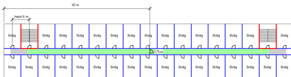
Figur 44 - illustration af referencebyggeriet, grøn farve angiver flugtvejsgang med mulighed for at flygte i to retninger, grå farve angiver områder med mulighed for at flygte i en retning.
