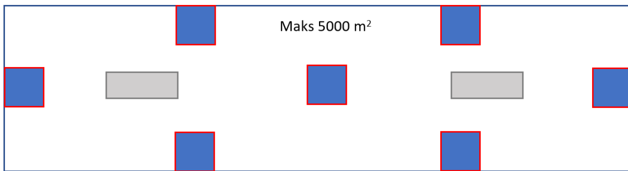
Figur 48 Principskitse af placeringen af brandsektioner og trapperum til indsats i referencebygningen. Brandsektioner er markeret med rødt, og de blå felter symboliserer en brandmandselevator samt en sikkerhedstrappe, de grå områder er de åbne forbindelser mellem to etager.
