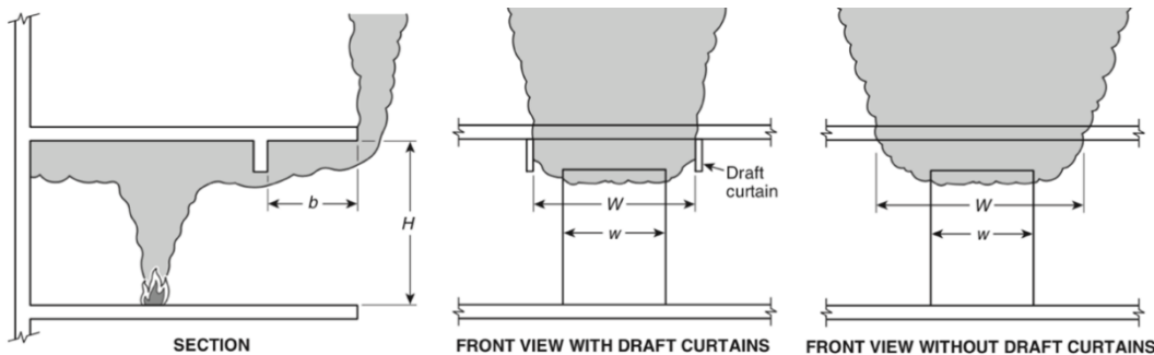
Figur 34: Illustration af en linjerøgfane
