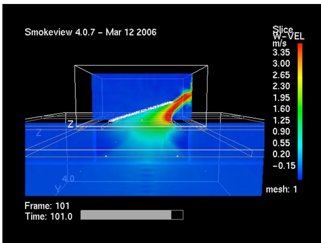
Figur 49: Fuld modellering af strømning igennem naturlig ventilationsåbning.
