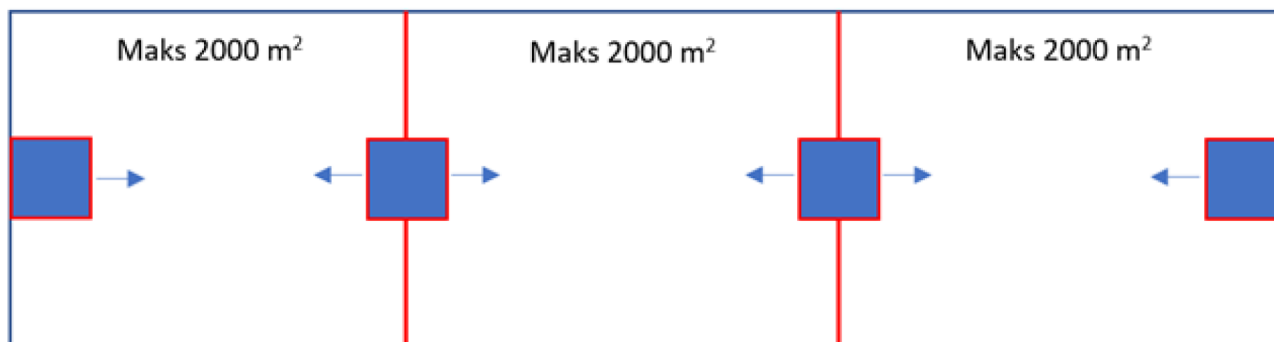
Figur 47 Principskitse af placeringen af brandsektioner og trapperum til indsats i analysebygningen. Brandsektioner er markeret med rødt, og de blå felter symboliserer en brandmandselevator samt en sikkerhedstrappe.
