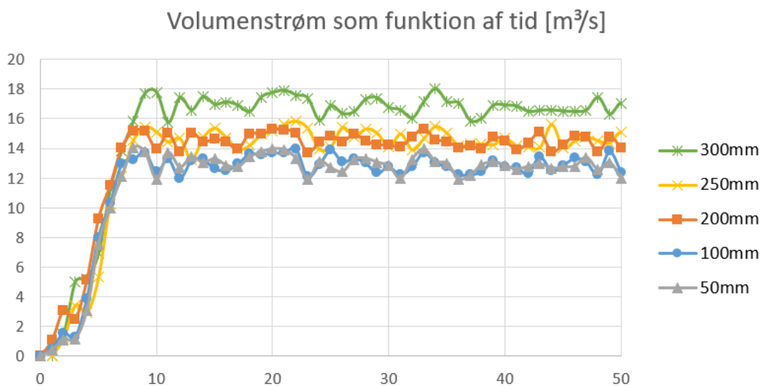
Figur 14: Eksempel på trinvis konvergens hvor resultaterne konvergerer parvist ved forøget finhed af beregningsnettet
