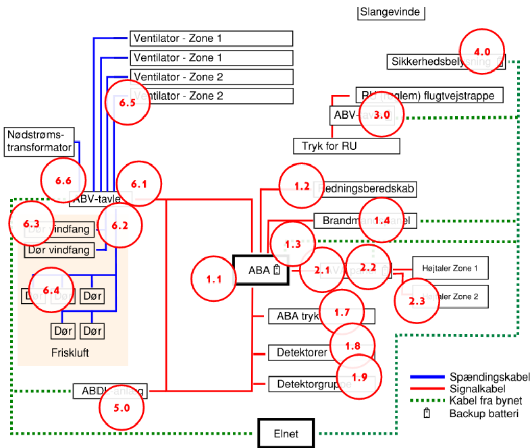
Figur 39: Diagrammatiske anlægsofbygning med angivelse af de identificerede svigt
