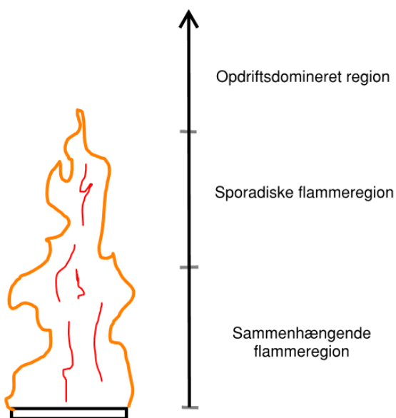
Figur 31: Regioner i McCaffrey røgfane.
