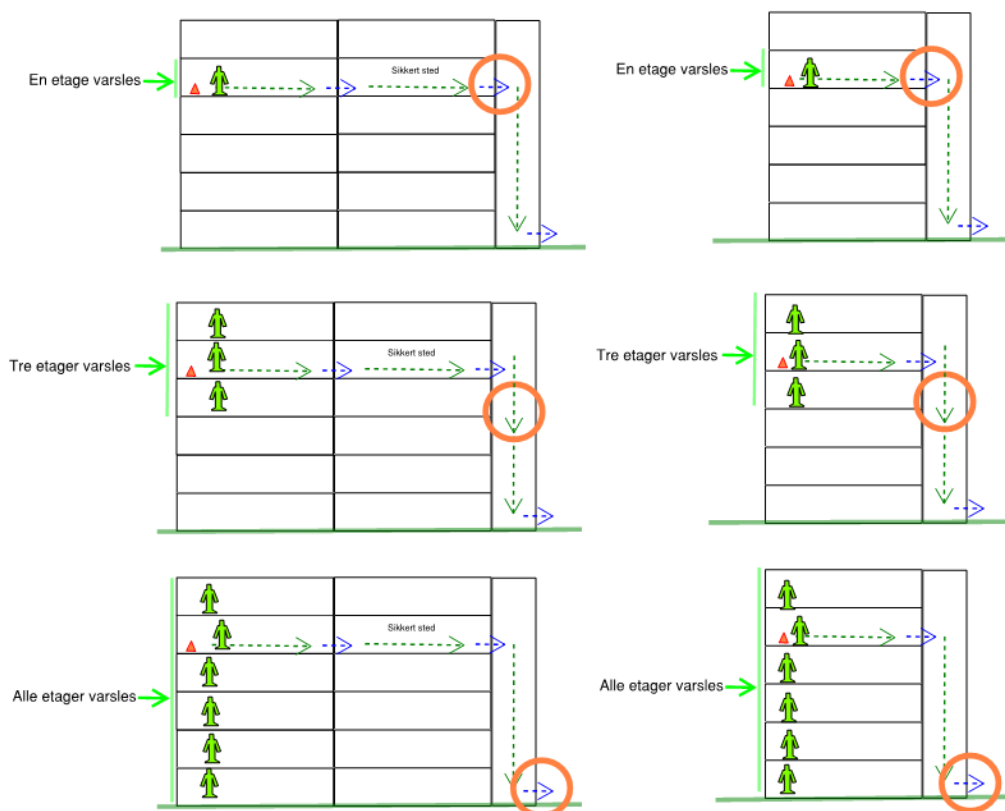
Figur 20: Eksempel på sidste flaskehals i kontorbygning ved forskellige varslingsscenerier for kontorbygning med evakuering via sikkert sted og direkte til flugtvejstrappe.
