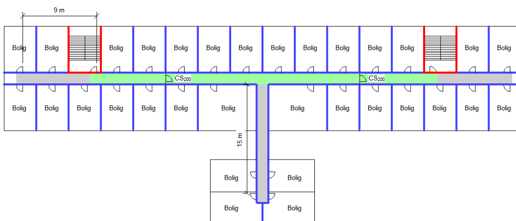
Figur 43 - illustration af analysebyggeriet, grøn farve angiver flugtvejsgang med mulighed for at flygte i to retninger, grå farve angiver områder med mulighed for at flygte i en retning.
