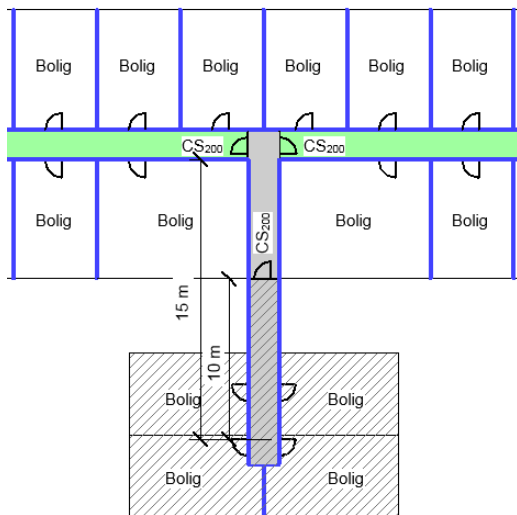
Figur 46 - illustration af analysebyggeriet med kompenserende tiltag. Grøn farve angiver flugtvejsgang med mulighed for at flygte i to retninger, grå farve angiver områder med mulighed for at flygte i en retning.
