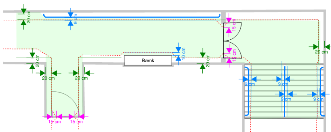
Figur 24 Eksempel på fastsættelse af effektiv bredde (rød stiple) i flugtvejssystem med vægge (med og uden håndlister), forhindringer og døre og trapper.
