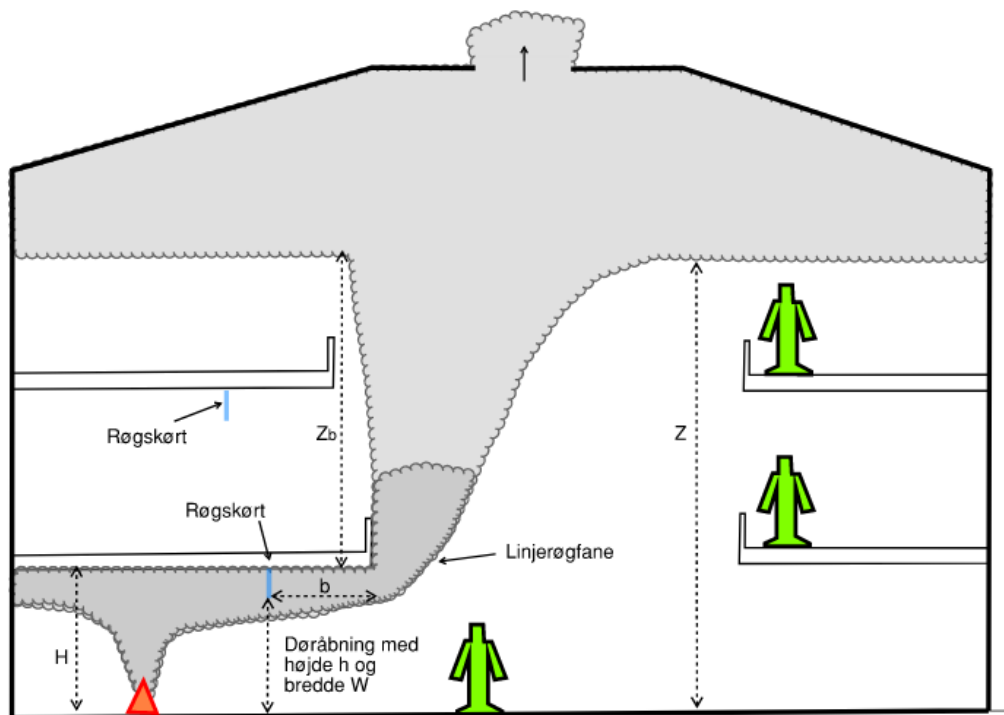
Figur 33: Linjerøgfane der viser røgspredning i et atrie
