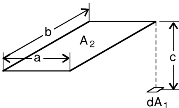
Figur 37: Synsfaktor mellem flade og punkt
