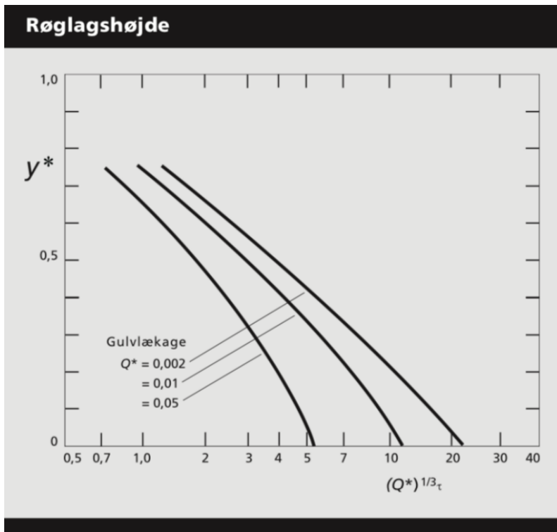
Figur 36: Røglagshøjden over gulv som funktion af tid - effekt, når højde, tid og effekt er normeret til dimensionsløse størrelser.
