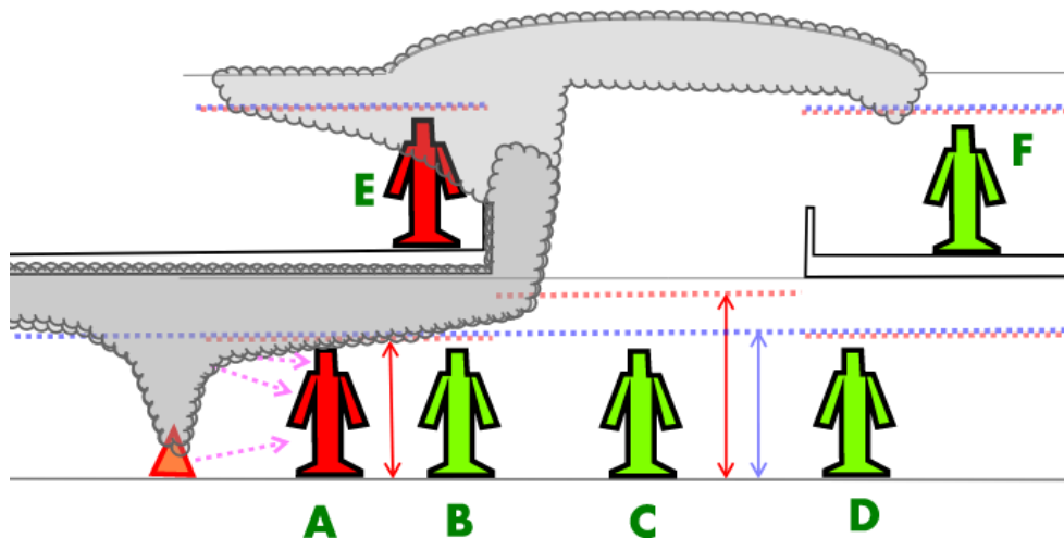
Figur 2: Lodret snit i indkøbscenter med seks områder, som evalueres i forhold til acceptkriterierne
