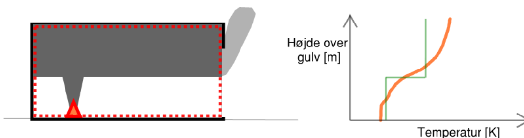
Figur 10: Princip for 2-zonemodellering med illustration af den forudsatte temperaturgradient (grøn) i den homogene øvre zone set i forhold til en virkelig temperaturgradient (orange).
