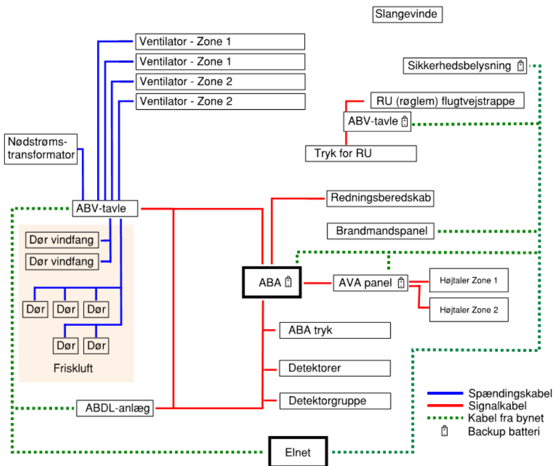
Figur 38: Diagrammatisk anlægsopbygning for brandsikringsanlæg
