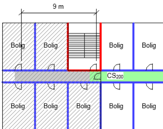
Figur 45 - illustration af analysebyggeriet med kompenserende tiltag, grøn farve angiver flugtvejsgang med mulighed for at flygte i to retninger, grå farve angiver områder med mulighed for at flygte i en retning. Skraveringen viser områder i røgzone, som direkte eller indirekte påvirkes af branden.
