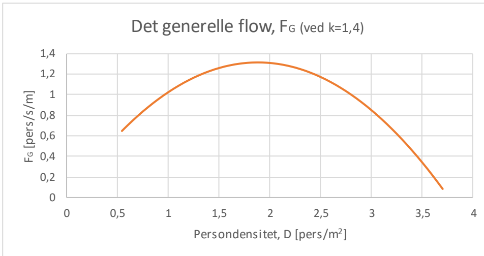
Figur 23: Kurve for generelt flow ved en k -værdi på 1,4 svarende til flow gennem døre, korridorer, døre og ramper
