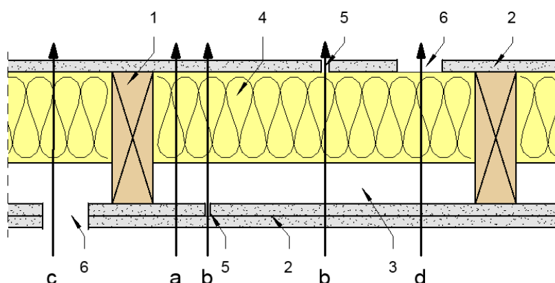
Figur 27 - Illustration af varmeovergangsveje i en lagopbygget bygningsdel
