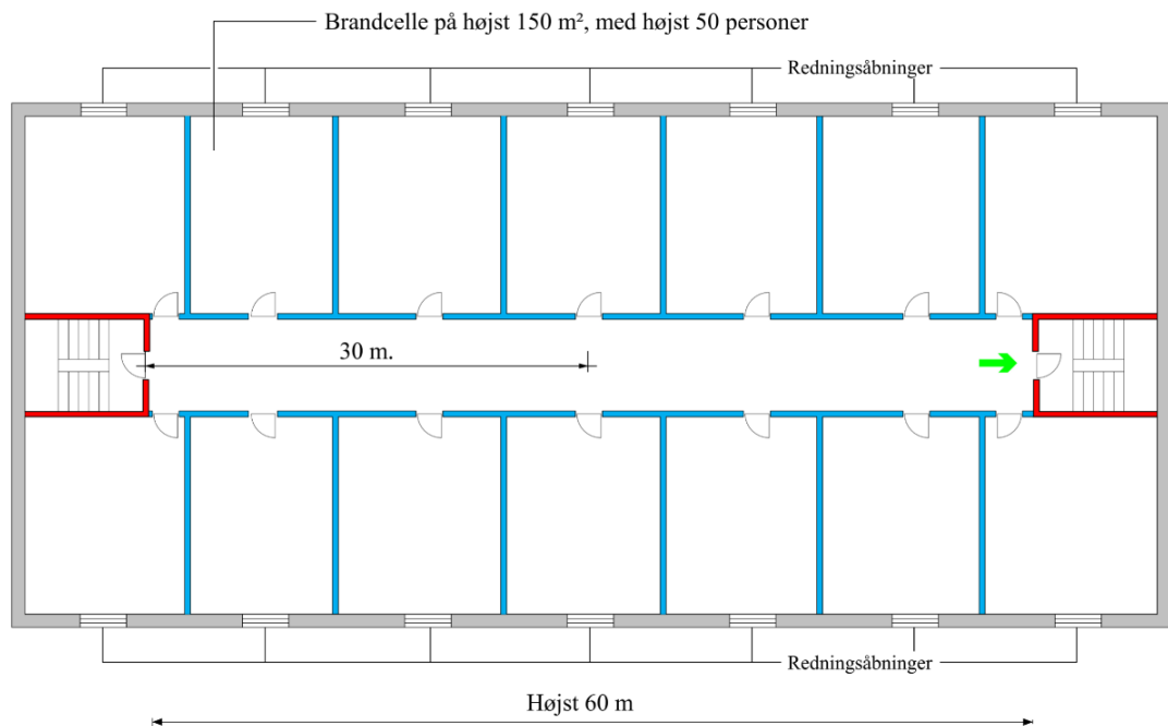
Figur 2.13. Placering af udgange fra flugtvejsgange.
