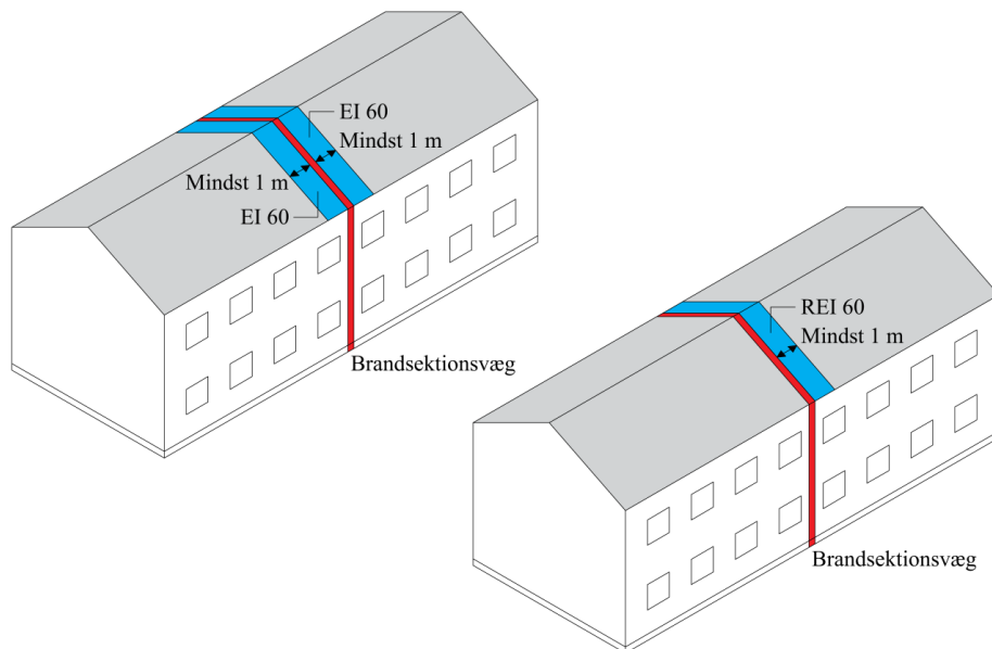
Figur 4.14. Brandkam og brandkammerstatning ved brandsektionsadskillelse for hindring af brandspredning over tag.
