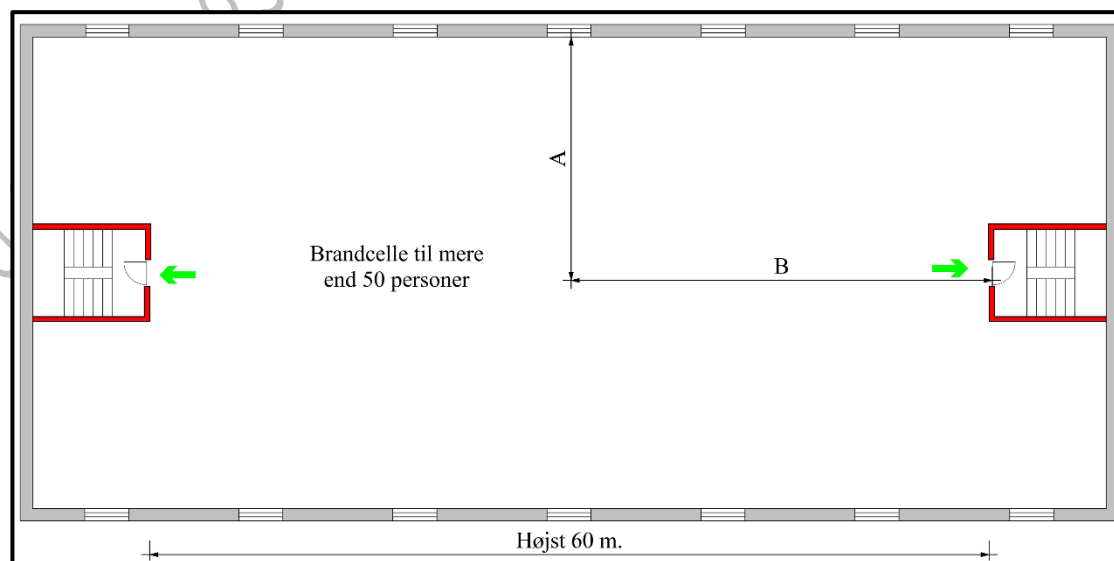
Figur 2.3.6 Døre til flugtveje fra brandcelle med flere end 50 personer, men færre end 150 personer.
