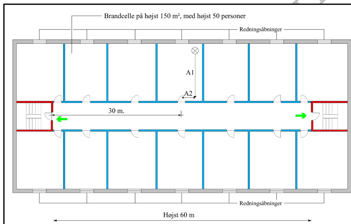
Figur 2.3.4 Døre til flugtveje fra brandcelle på højst 150 m 2 og med højst 50 personer.
