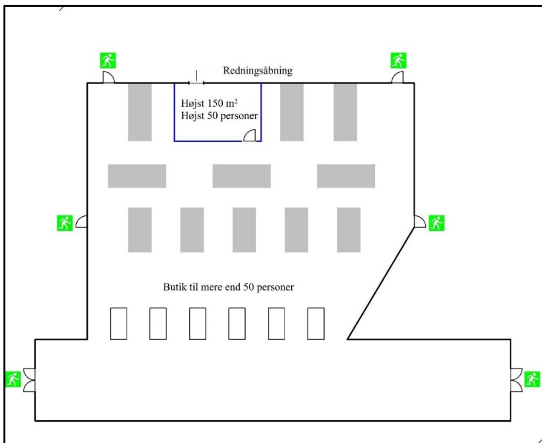
Figur 2.3.5 Udgang fra en indeliggende brandcelle via en anden brandcelle.
