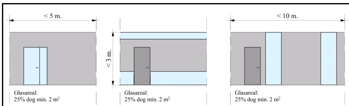
Figur 2.3.12 Præ-accepteret løsning på fordeling af gennemsigtigt glas (blå farve) uden afdækning for forskellige konfigurationer.
