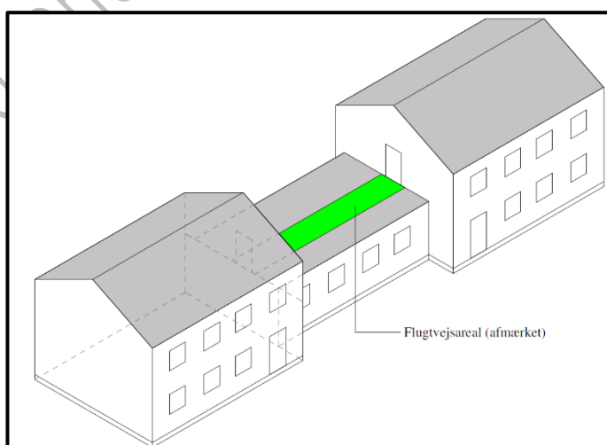
Figur 2.3.20 Flugtvej over tag til højst 50 personer.
