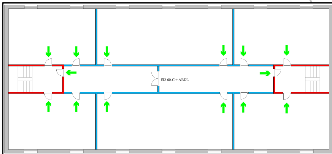
Figur 2.3.7 Opdeling af flugtvejsgang for etablering af uafhængige flugtveje fra opholdsrum.
