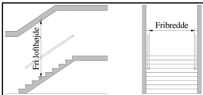
Figur 2.3.22 Definition af en trappes geometri.
