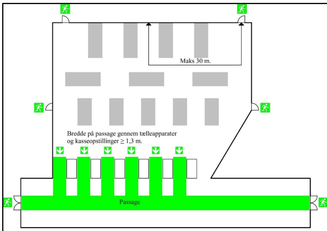
Figur 2.3.9 Præ-accepteret løsning for flugtveje fra butik med kasseopstilling. Passager (grøn markering) udføres med en fri bredde på minimum 1,3 m. Primære flugtvejsdøre skal mindst være 1,2 m i fri bredde.
