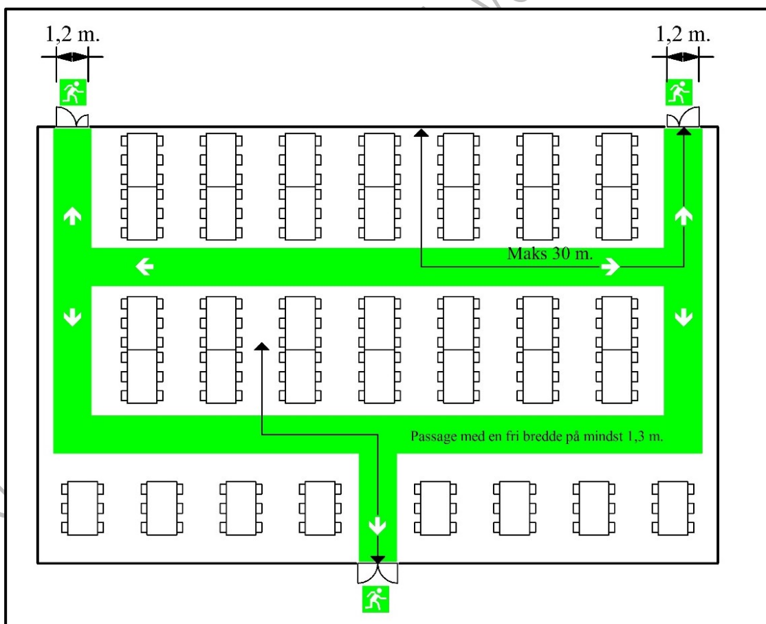
Figur 2.3.8 Præ-accepteret løsning for forsamlingslokale med passager på mindst 1,3 m fri bredde.
