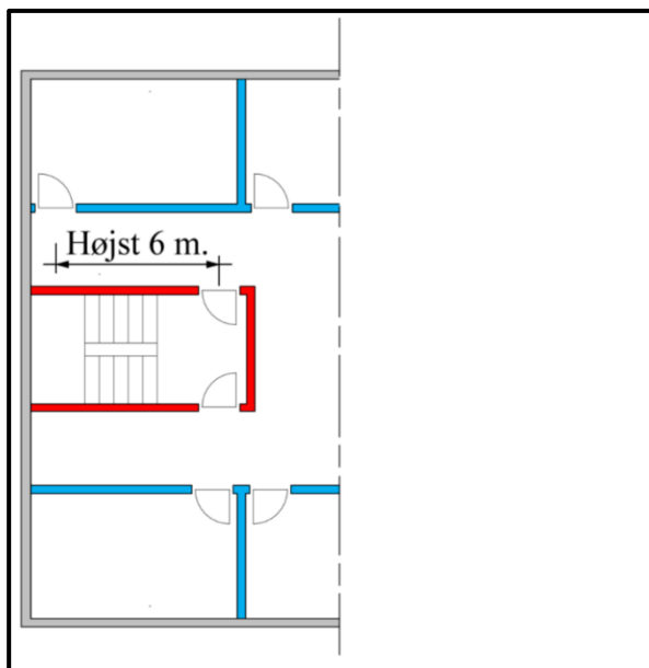
Figur 2.3.17 Udgang i én retning i en flugtvejsgang.
