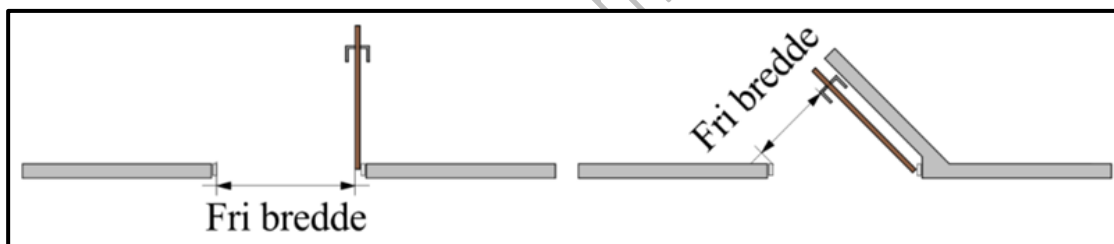
Figur 2.3.14 Måling af en dørs frie bredde ved henholdsvis en åbning på 90° og ved åbning på mindre end 90°.
