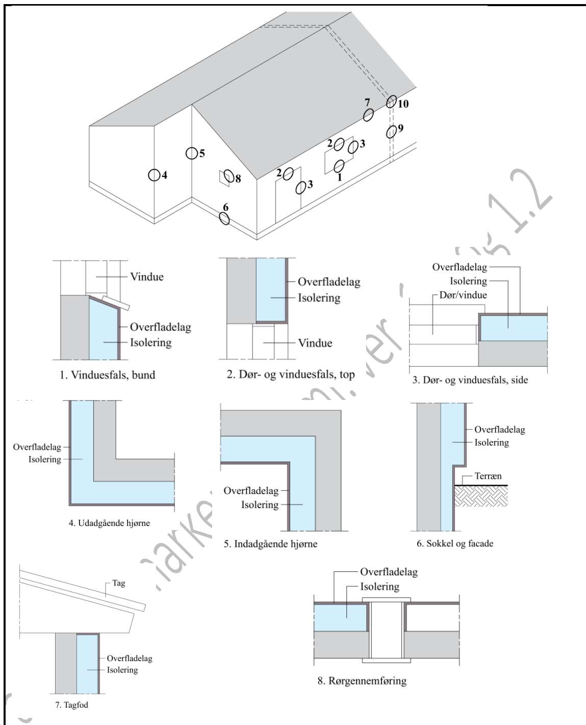
Figur 4.2.3 Præ-accepterede løsninger, hvor det er vigtigt at sikre, at overfladelag (inddækningen) af isoleringsmaterialet, som ikke mindst er materiale klasse D-s2,d2 [klasse B materiale], er korrekt udført.
