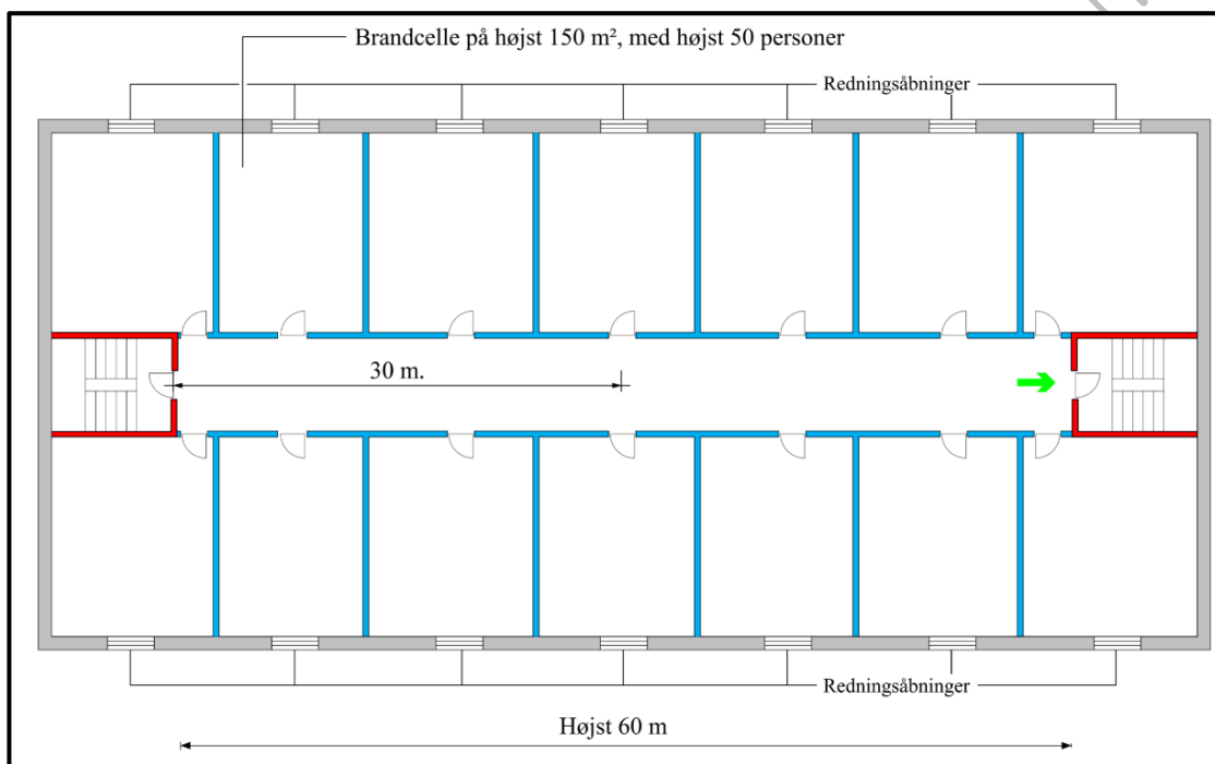
Figur 2.3.16 Placering af udgange fra flugtvejsgange.
