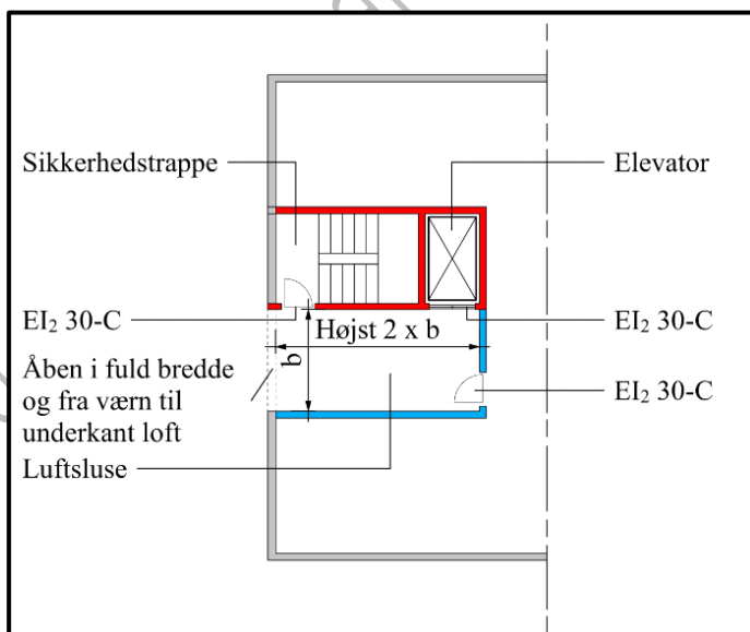
Figur 2.3.23 Princip for udførelse af luftsluse placeret over terræn for bygninger med gulv i øverste etage højst 22 meter over terræn.
