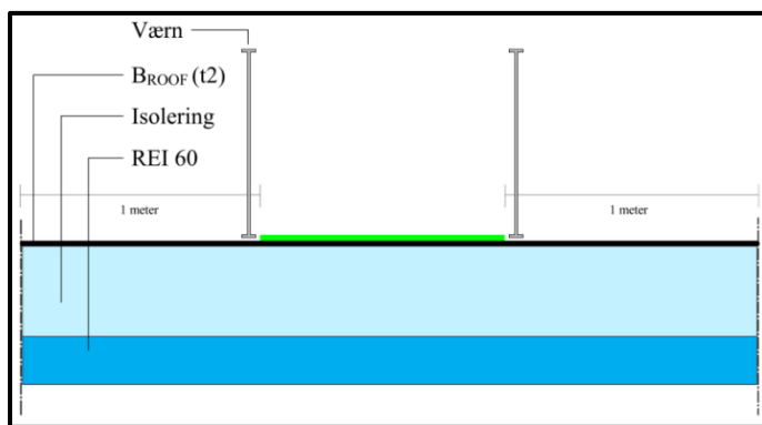
Figur 2.3.21 Brandmæssig adskillelse under flugtvej over tag. Der må ikke etableres åbninger eller gennemføringer i en afstand af mindst 1,0 m fra kanten af flugtvejen.
