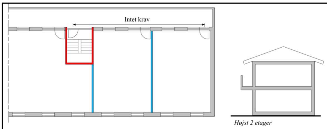
Figur 2.3.14 Adgang til flugtvejstrappe via altangang for bygning med højst 2 etager over terræn og redningsberedskabet kan nå altangangen med deres bærbare stiger.
