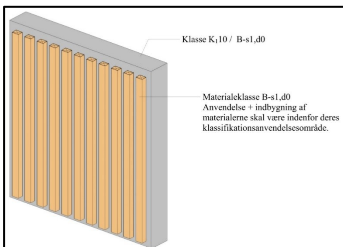
Figur 4.2.18 Præ-accepteret løsning på indvendig komplettering i form af listeværk på indvendig beklædning mindst klasse K_1 10 / B-s1, d0 [klasse 1 beklædning].
