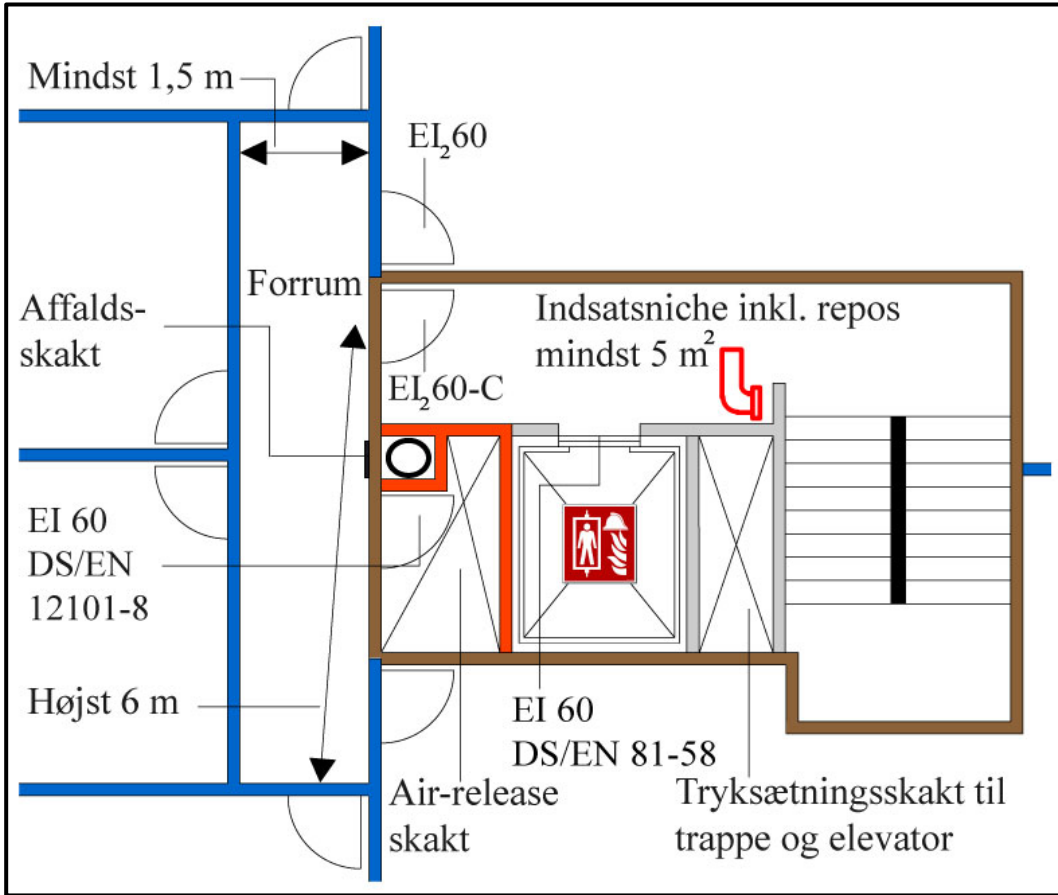
Figur 05.09.02: Præ-accepteret tryksat trapperum nr. 02
