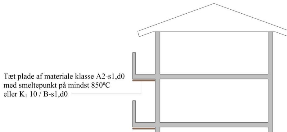
Figur 10 Altan som ikke mindst er materiale klasse A2-s1,d0 skal sikres mod brandspredning fra underliggende etage.
