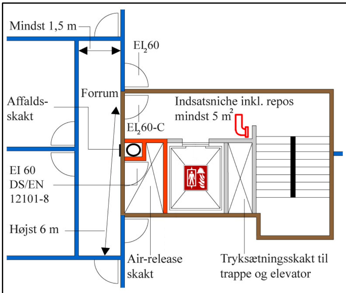
Figur 5.9.2 Præ-accepteret tryksat trapperum nr. 02
