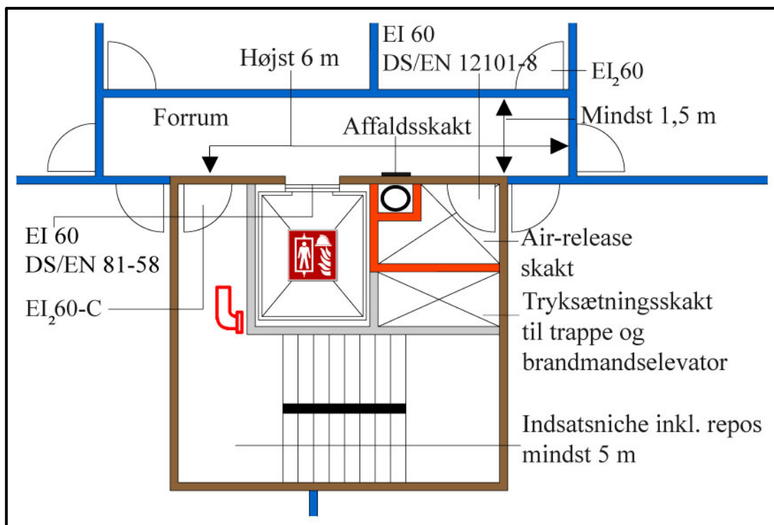
Figur 5.9.4 Præ-accepteret tryksat trapperum nr. 04.
