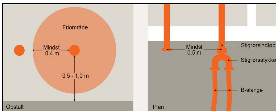
Figur 5.14.2 Placering af stigrørsindløb.
