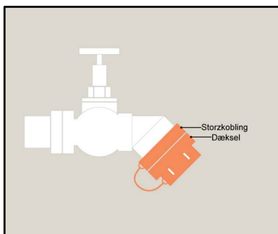
Figur 5.14.5 Stigrørsudtag med afspærringsventil.
