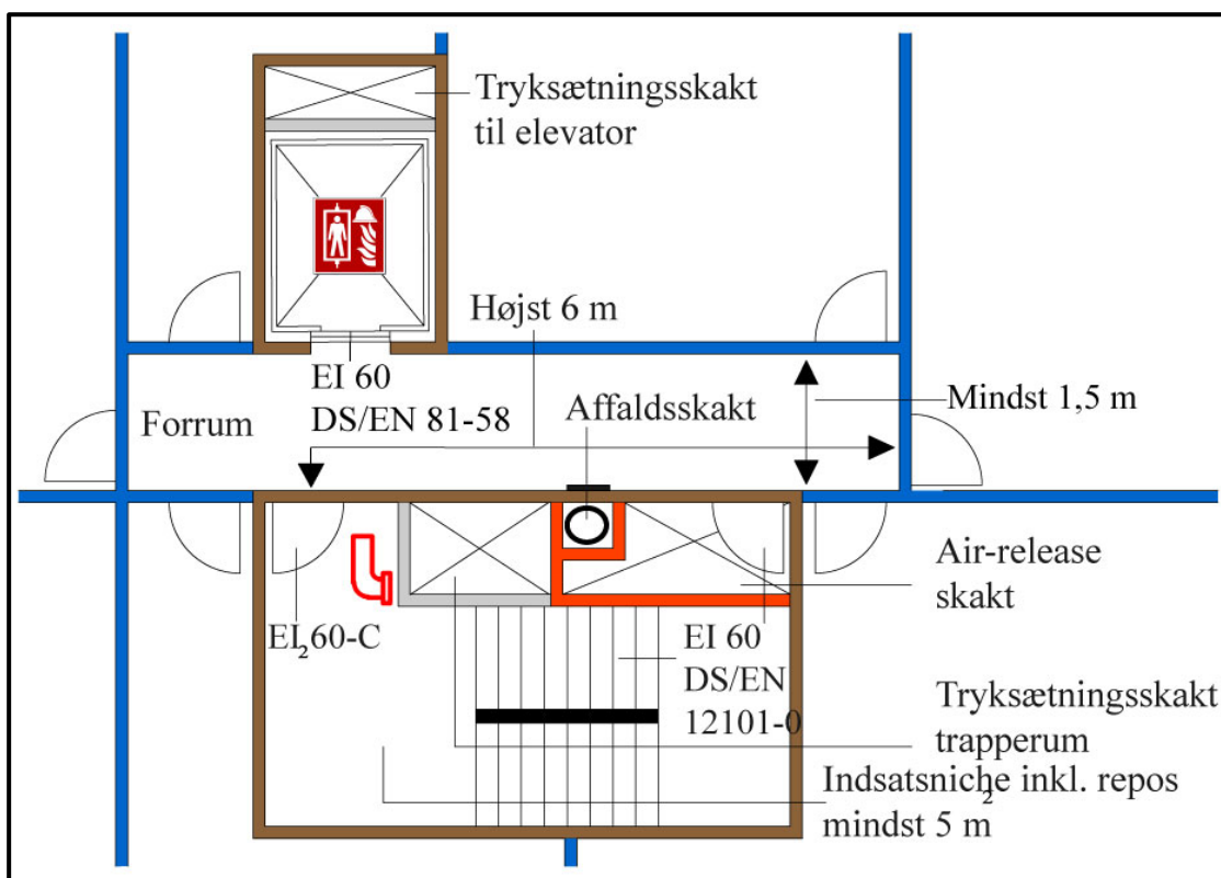
Figur 5.9.3 Præ-accepteret tryksat trapperum nr. 03.
