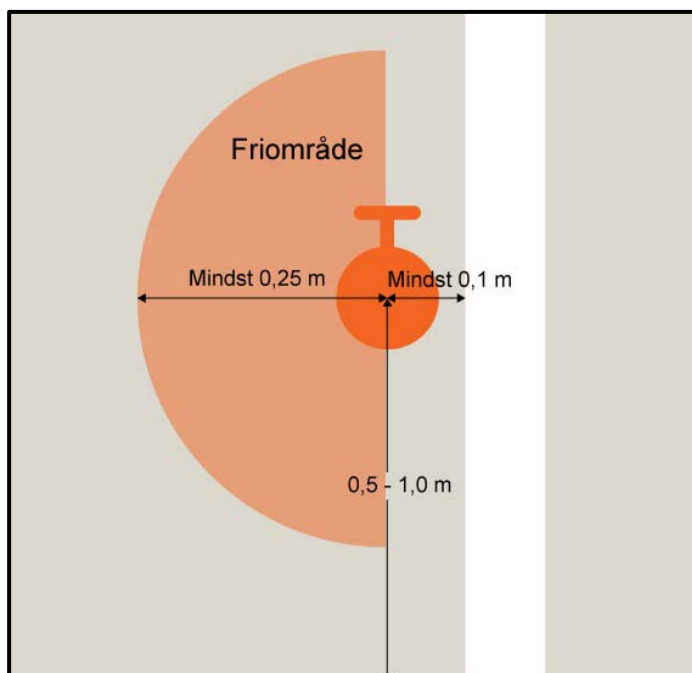
Figur 5.14.4 Stigrørsudtag med friområde.
