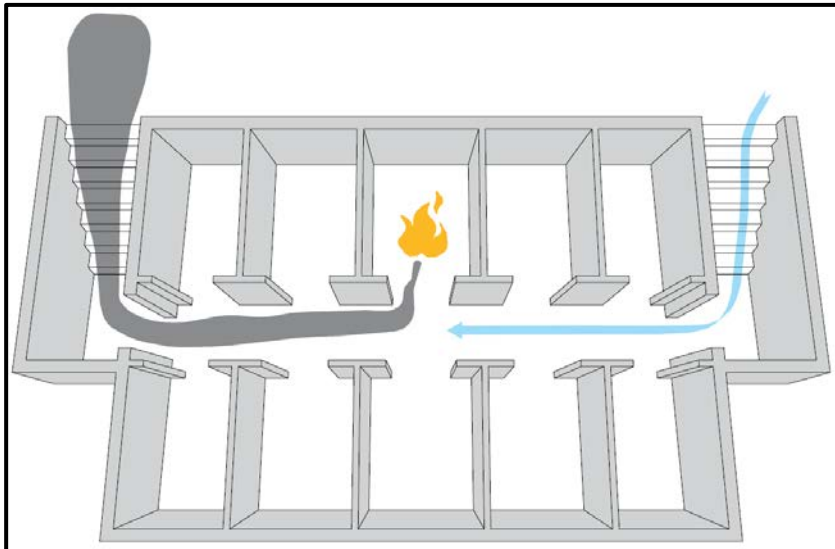
Figur 5.11.3 Eksempel på tværv ventilation.
