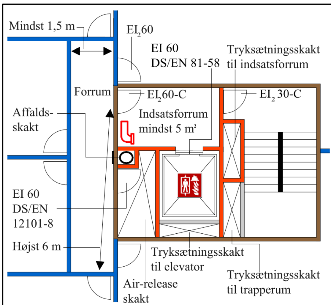
Figur 5.9.1 Præ-accepteret tryksat trapperum nr. 01.
