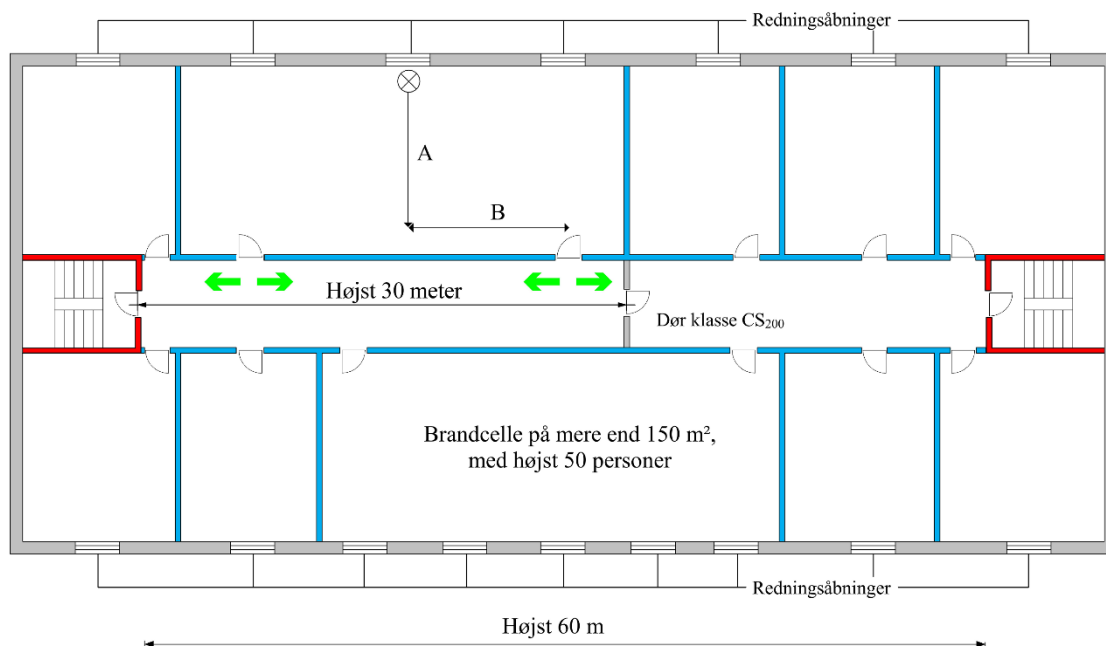
Figur 2.3. Døre til flugtveje fra brandceller større end 150 m 2 og med højst 50 personer.
