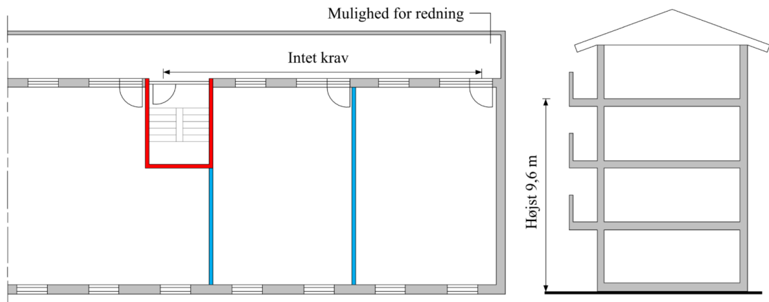
Figur 2.13. Adgang til flugtvejstrappe via altangang for bygning, hvor gulv i øverste etage er højst 9,6 meter over terræn og redningsberedskabet kan nå altangangen med deres bærbare stiger.
