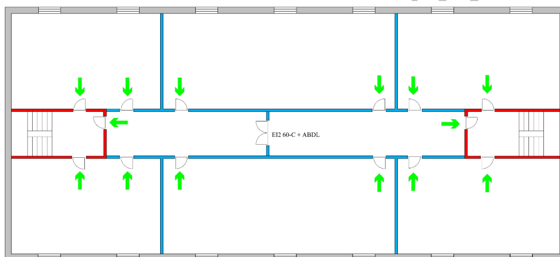
Figur 2.5. Opdeling af flugtvejsgang for etablering af uafhængige flugtveje fra opholdsrum.
