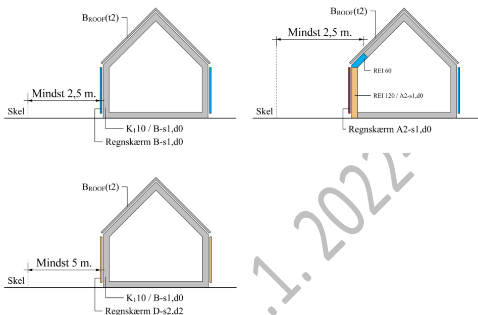
Figur 4.1 Afstande til skel mod nabo, vej- og stimidte fra bygningen ift. udvendige vægoverflader og tagdækning.
