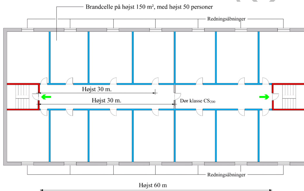
Figur 2.10. Placering af udgange fra flugtvejsgange.
