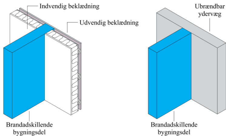
Figur 4.11 Sammenbygning af facade og brandadskillende bygningsdel, hvor den brandadskillende væg føres frem til indersiden af den udvendige beklædning. Samme princip gælder for etageadskillelse.
