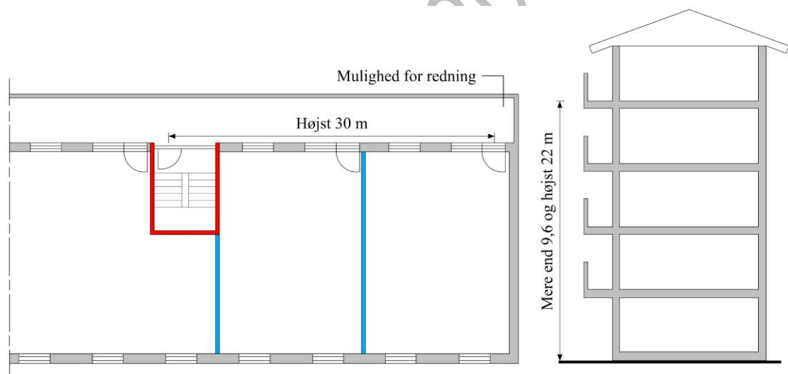
Figur 2.14. Adgang til flugtvejstrappe via altangang for bygning, hvor gulv i øverste etage er mellem 9,6 og højst 22 meter over terræn og redningsberedskabet kan nå enden af altangangen med deres kørbare stiger.
