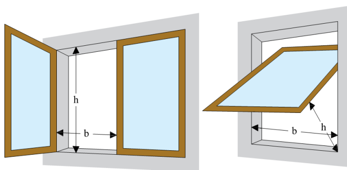
Figur 2.20. Udformning af redningsåbning til personredning.
