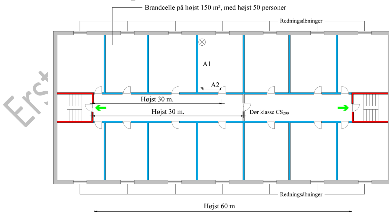
Figur 2.4. Døre til flugtveje fra brandcelle på højst 150 m 2 og med højst 50 personer.
