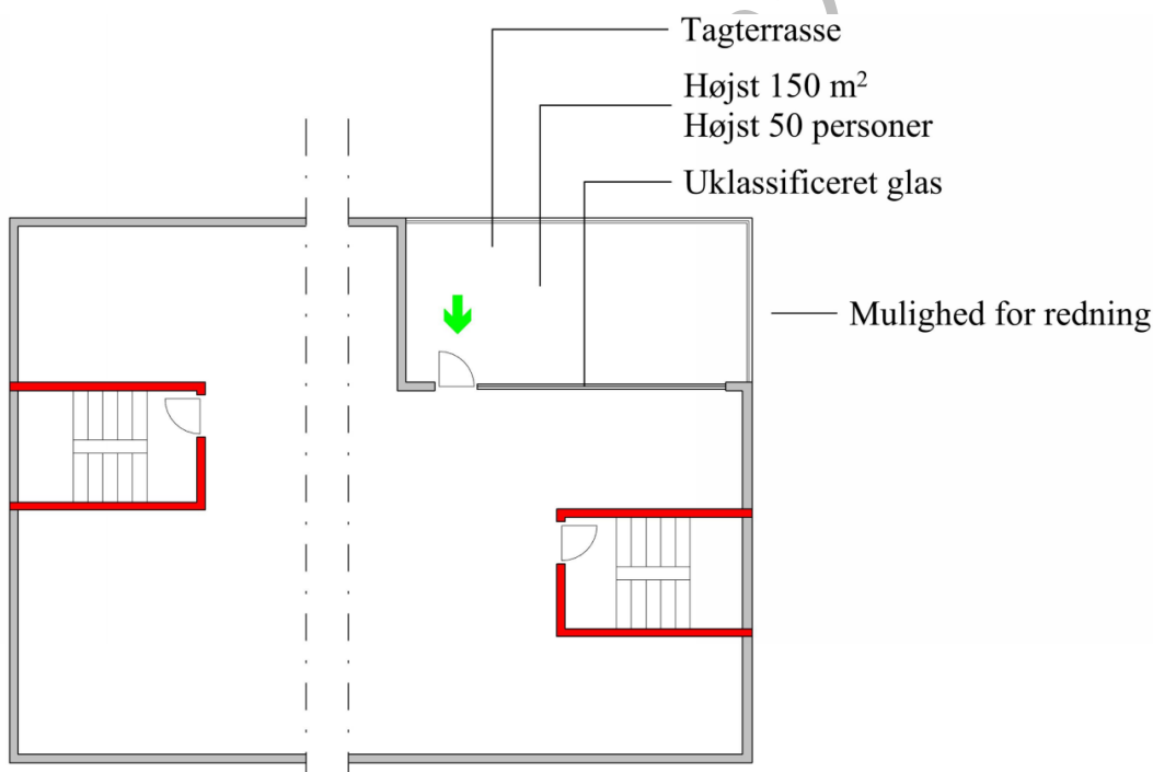
Figur 2.6. Flugtvej fra tagterrasse for bygninger, hvor gulv i øverste etage er højst 9,6 meter over terrænen.
