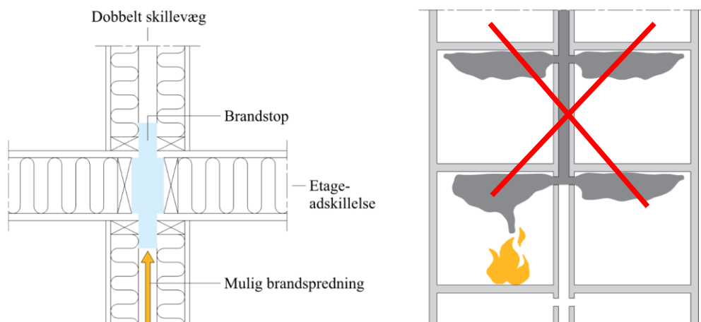
Figur 4.19 Brandstop mellem brandmæssige enheder
