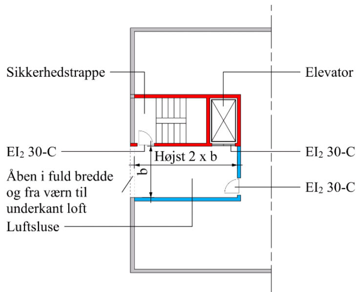
Figur 2.19. Princip for udførelse af luftsluse placeret over terræn for bygninger med gulv i øverste etage højst 22 meter over terræn.
