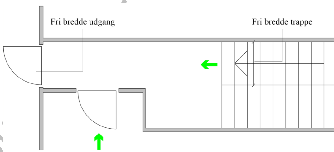
Figur 2.9. Fri bredde for udgang til det fri fra trapperum.
