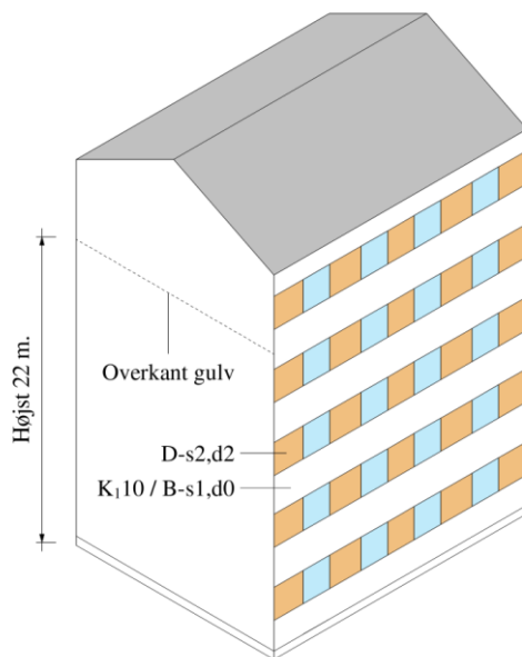
Figur 4.5 Præ-accepteret løsning på mindre dele af ydervæggens areal udført med regnskærm, mindst som materiale klasse D-s2,d2 [klasse B materiale]. Det samlede areal må højst udgøre 20% af ydervæggens areal.
