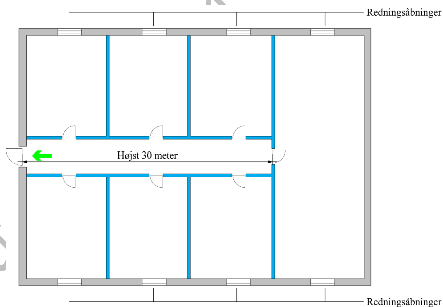
Figur 2.12 Udgang i én retning i en flugtvejsgang, med underkant af redningsåbninger mindre end 2,0 m over terræn.
