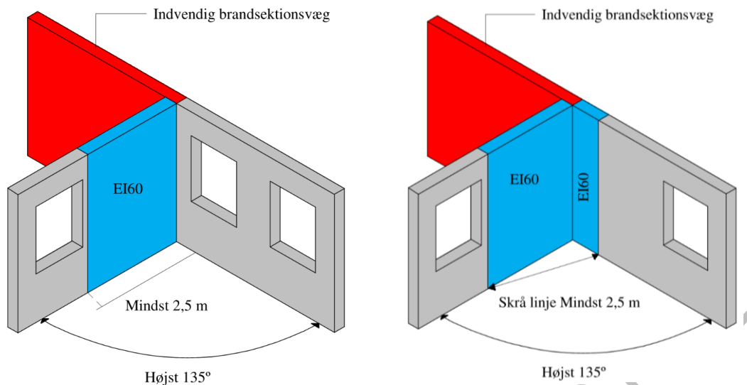
Figur 4.12 Sikring af vandret brandspredning/vinkelsmitte ved brandsektionsafgrænsende vægge.
