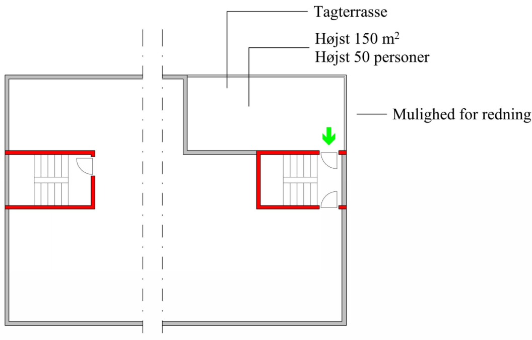
Figur 2.7. Flugtvej fra tagterrasse for bygninger, hvor gulv i øverste etage er højst 22 meter over terræn
