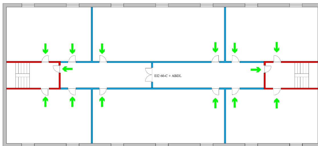
Figur 2.5. Opdeling af flugtvejsgang for etablering af uafhængige flugtveje fra opholdsrum.
