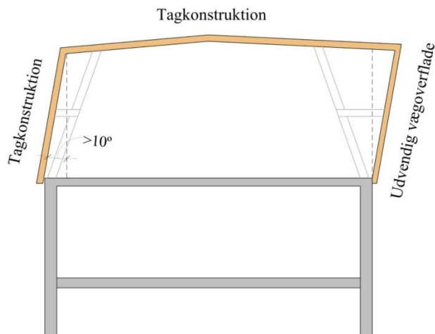
Figur 4.6 Definition af skrående facade som hhv. udvendig vægoverflade og tagkonstruktion, gældende for øverste etage.
