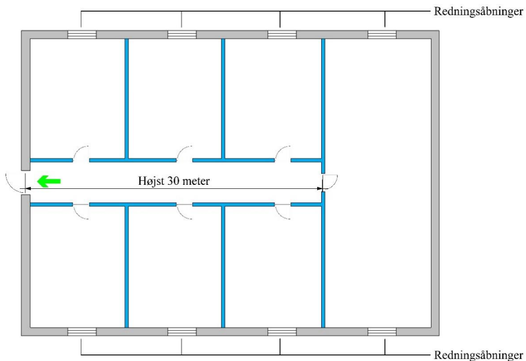
Figur 2.17 Udgang i én retning i en flugtvejsgang, med underkant af redningsåbninger mindre end 2,0 m over terræn.
