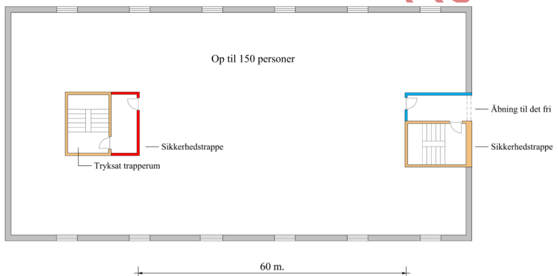
Figur 2.25. Bygningsafsnit med op til 150 personer, hvor der er adgang til 2 sikkerhedstrapper, hvor gulv i øverste etage er mere end 22 meter og højst 45 meter over terræn.
