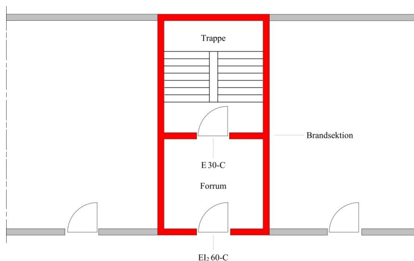
Figur 4.17. Præ-accepteret løsninger på en trappe som er ført til kælder i en kontorbygning, hvor gulv i øverste etage er højst 22 meter over terræn.
