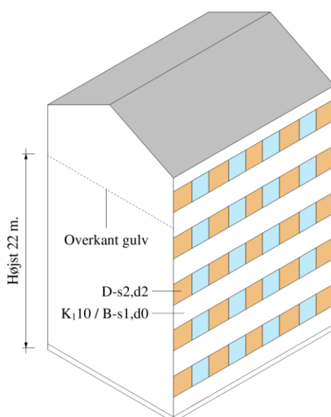
Figur 4.5 Præ-accenteret løsning på mindre dele af ydervæggens areal udført med regnskærm, mindst som materiale klasse D-s2,d2 [klasse B materiale]. Det samlede areal må højst udgøre 20 % af ydervæggens areal.
