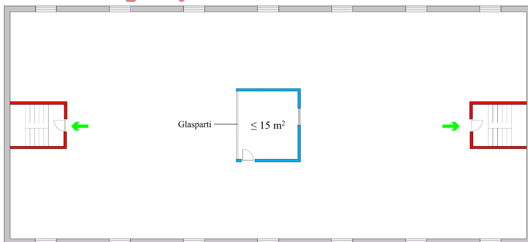
Figur 4.21. Enkeltstående kontor/mødelokale på maksimalt 15 m 2 udføres med brandteknisk uklassificerede glaspartier mod omgivende opholdsrum/flugtvejsareal, med visuel kontakt.
