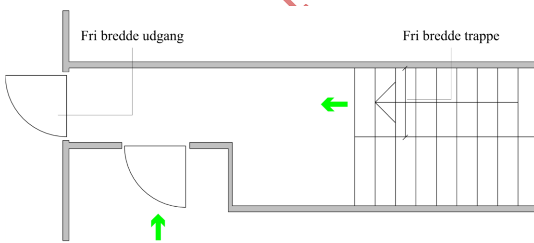
Figur 2.14. Fri bredde for udgang til det fri fra trapperum.
