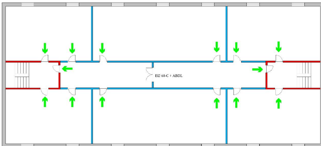
Figur 2.8. Opdeling af flugtvejsgang for etablering af uafhængige flugtveje fra opholdsrum.
