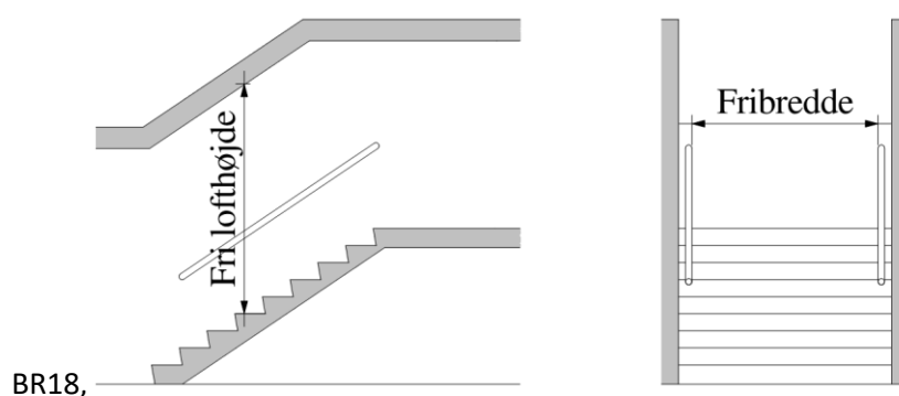
Figur 2.23. Definition af en trappes geometri.
