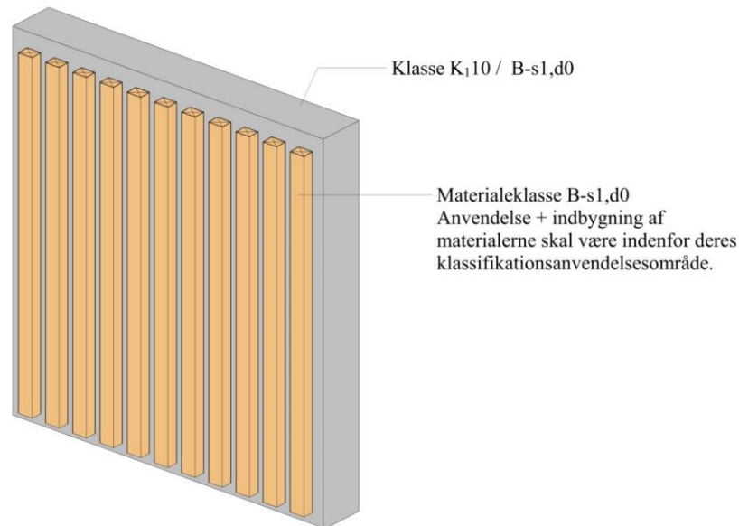
Figur 4.24. Præ-accepteret løsning på indvendig komplettering i form af listeværk på indvendig beklædning mindst klasse K 1 10 / B-s1,d0 [klasse 1 beklædning].
