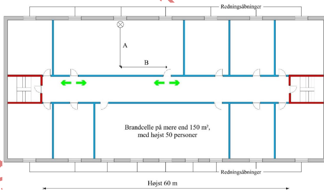
Figur 2.3. Døre til flugtveje fra brandceller over 150 m 2 og med højst 50 personer.
