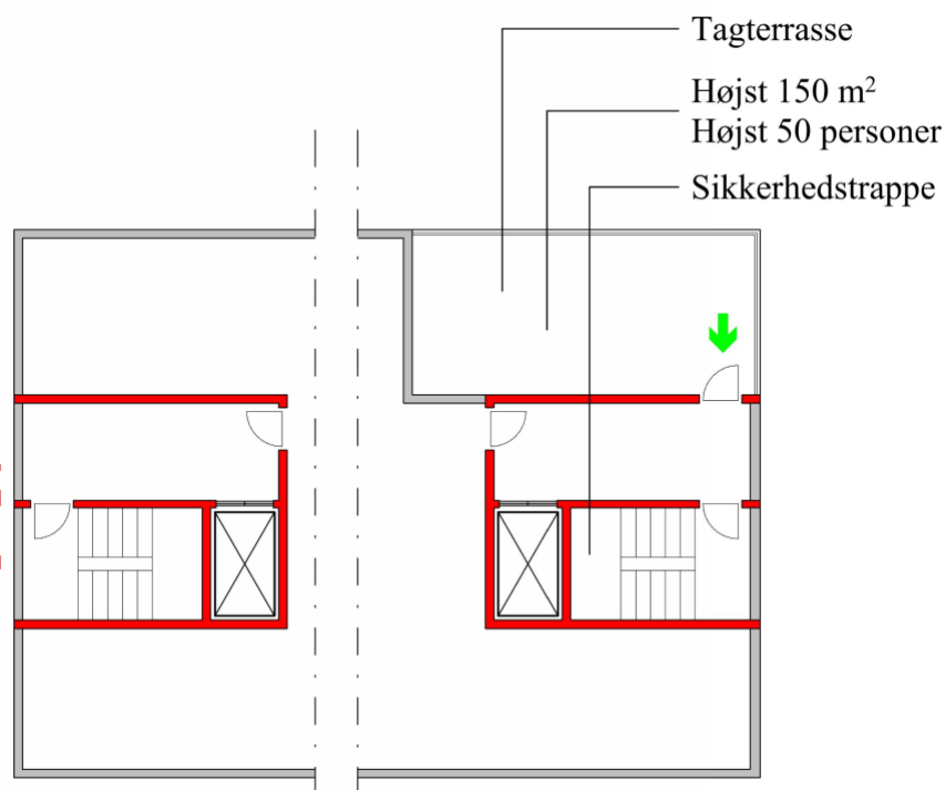
Figur 2.12. Flugtvej fra tagterrasse for bygninger, hvor gulv i øverste etage er mere end 22 meter over terræn og højst 45 meter over terræn.
