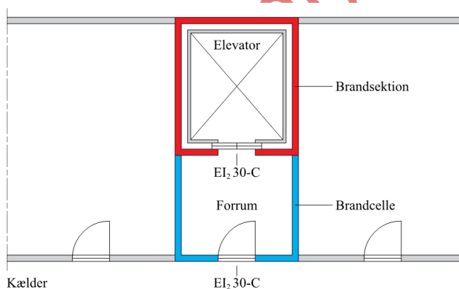
Figur 4.18. Adgang til kælderen via forrum fra elevator.
