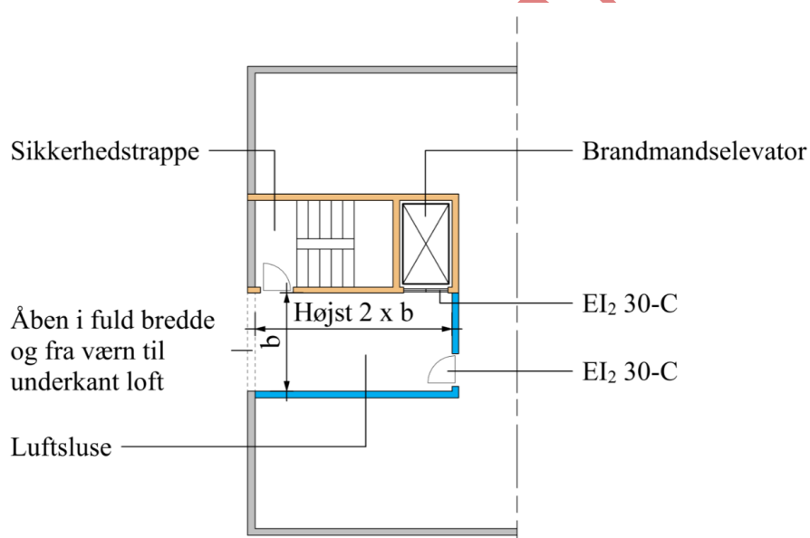
Figur 2.24. Princip for udførelse af luftsluse placeret over terræn for bygninger med gulv i øverste etage mere end 22 meter over terræn og højst 45 meter over terræn.
