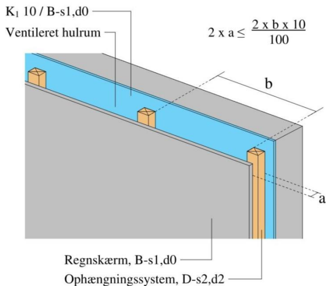
Figur 4.8. Beregningsmetode til den frie overflade for en regnskærms ophængningssystem. Alle klassifikationer er minimumskrav.
