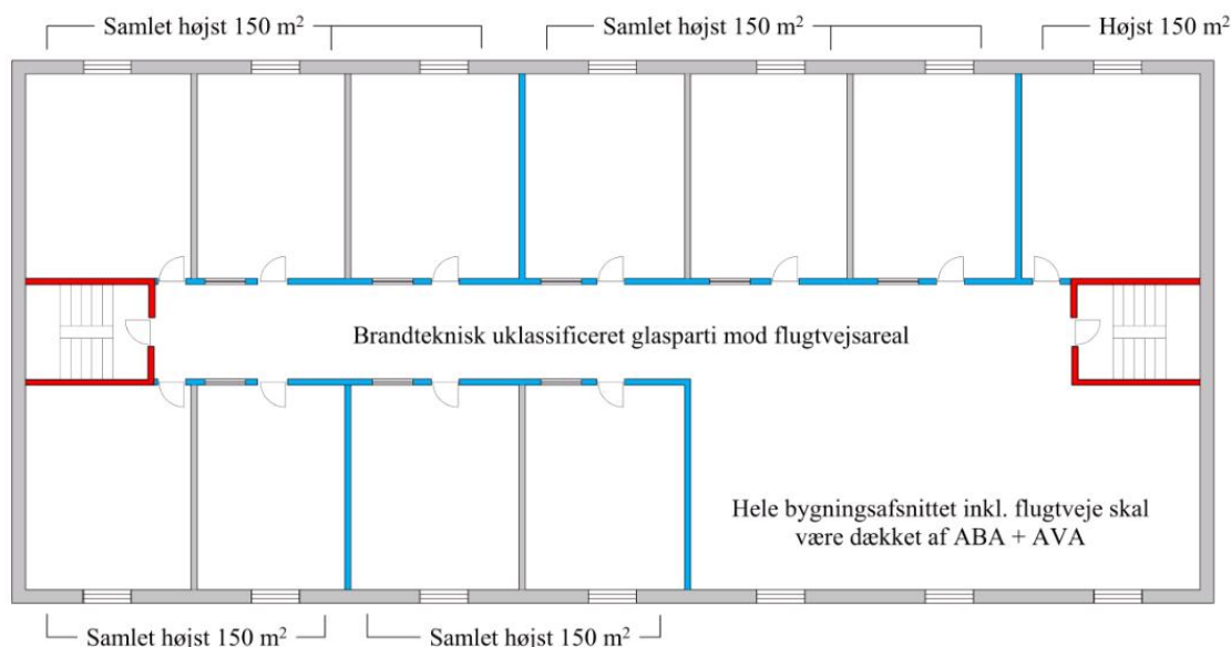
Figur 4.20. Præ-accepteret løsning på brandteknisk uklassificerede glasadskillelser mellem opholdsrum og flugtvejsareal. Bygningsafsniitet inklusive tilhørende flugtveje er udført med ABA og AVA.
