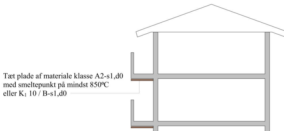
Figur 4.9 Altan som ikke mindst er materiale klasse A2-s1,d0 skal sikres mod brandspredning fra underliggende etage.
