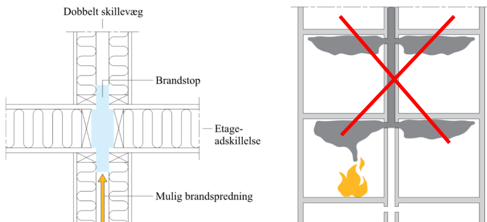
Figur 4.23 Brandstop mellem brandmæssige enheder
