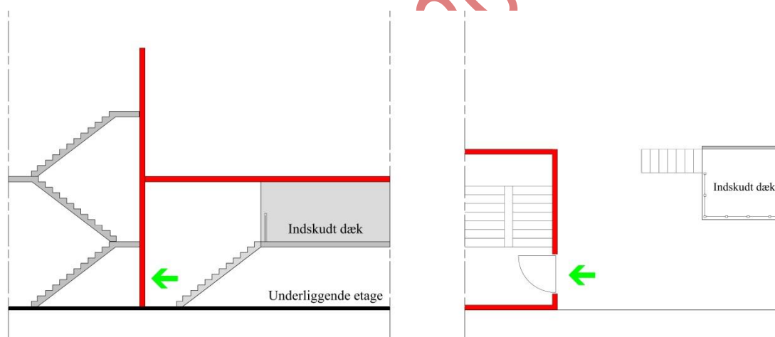
Figur 2.9. Flugtvejsprincip fra en brandcelle med et indskudt dæk og hvor der ikke er adgang til flugtvejstrappe fra begge etager.
