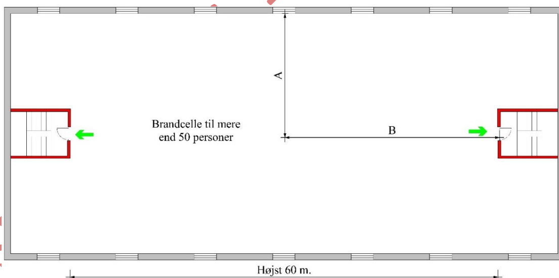
Figur 2.7. Døre til flugtveje fra brandcelle med mere end 50 personer, men mindre end 150 personer.
