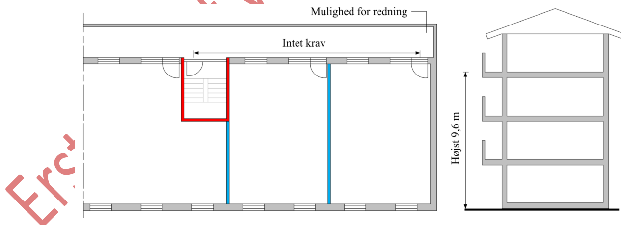
Figur 2.18. Adgang til flugtvejstrappe via altangang for kontorbygning, hvor gulv i øverste etage er højst 9,6 meter over terræn og redningsberedskabet kan nå altangangen med deres bærbare stiger.
