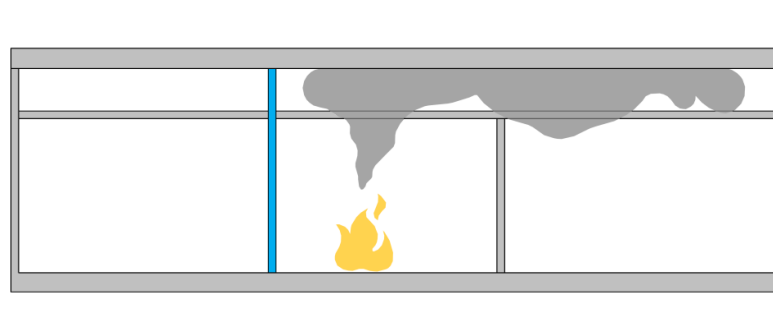
Figur 4.25. Kun brandklassificerede vægge føres op gennem nedhængt loft til underside af overliggende etage eller tagkonstruktion.
