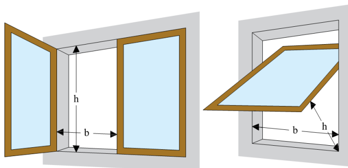
Figur 2.28. Udformning af redningsåbning til personredning.
