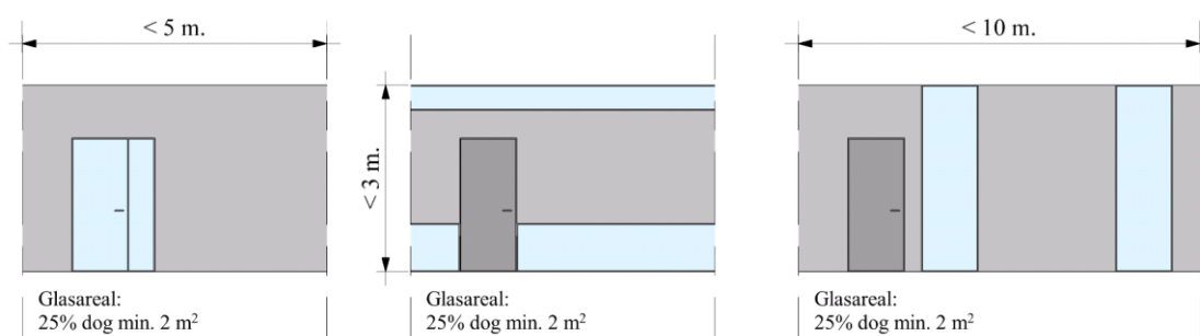
Figur 4.22. Præ-accepteret løsning på fordeling af gennemsigtigt glas (blå farve) uden afdækning for forskellige konfigurationer.
