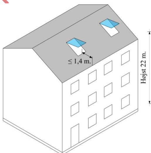
Figur 2.29. Udformning af redningsåbning i tagflade
