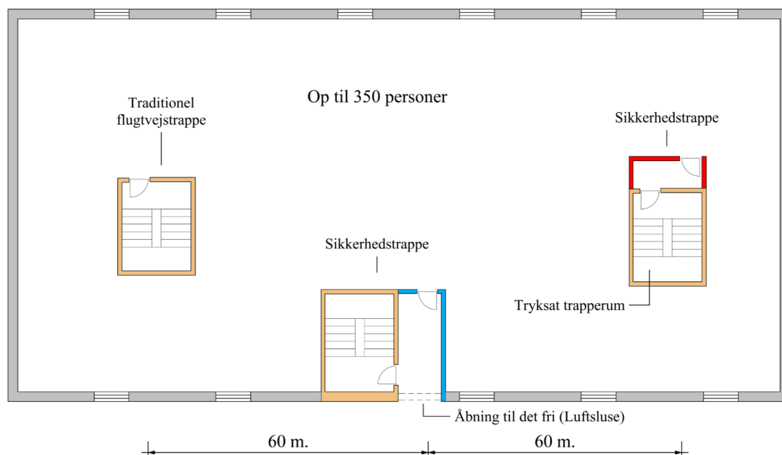
Figur 2.26. Præ-accepteret løsning på bygningsafsnit med op til 350 personer, hvor der er adgang til 2 sikkerhedstrapper og 1 traditionel flugtvejstrappe, i bygninger hvor gulv i øverste etage er mere end 22 meter og højst 45 meter over terræn.
