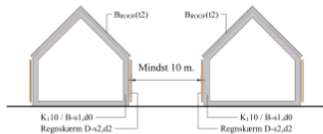
Figur 4.2 Afstand mellem bygninger på samme grund ift. udvendige vægoverflader. Alle klassifikationer er minimumskrav.
