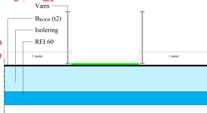
Figur 2.22. Brandmæssig adskillelse under flugtvej over tag. Der må ikke etableres åbninger eller gennemføringer i en afstand af min. 1 meter fra kanten af flugtvejen.
