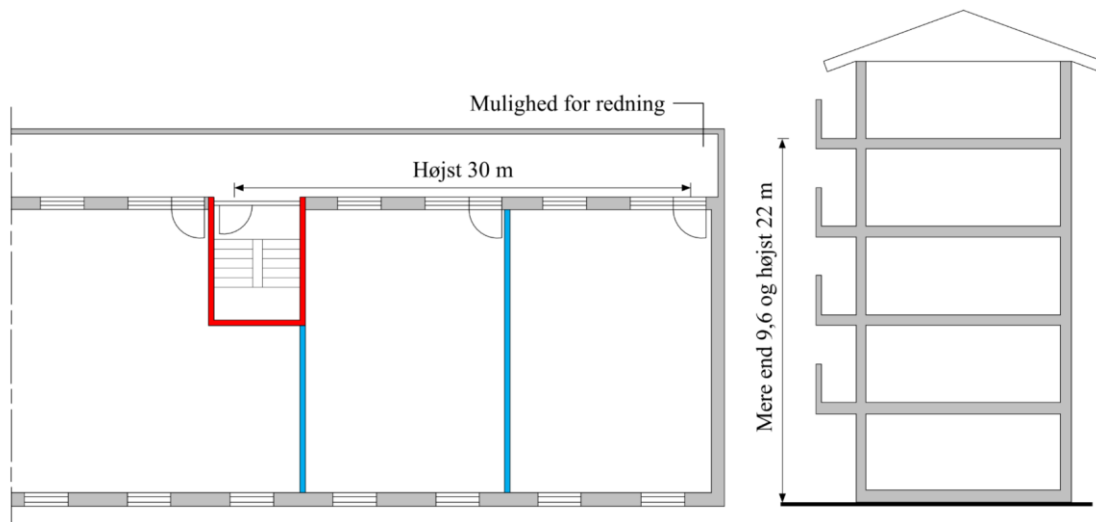
Figur 2.19. Adgang til flugtvejstrappe via altangang for kontorbygning, hvor gulv i øverste etage er mellem 9,6 og 22 meter over terræn og redningsberedskabet kan nå enden af altangangen med deres kørbare stiger.
