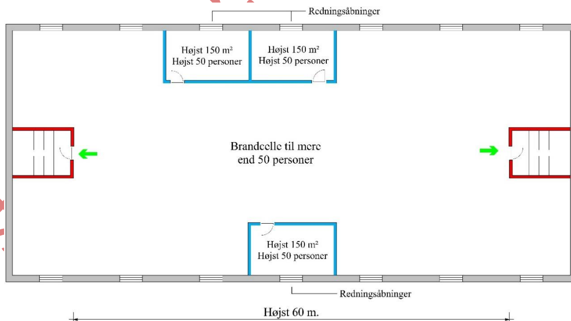
Figur 2.5. Udgang fra en indeliggende brandcelle via en anden brandcelle.
