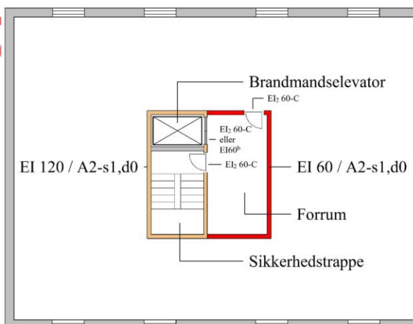
Figur 2.27. Placering af brandmandselevator ift. sektioner og døre samt klassifikation af døre.
