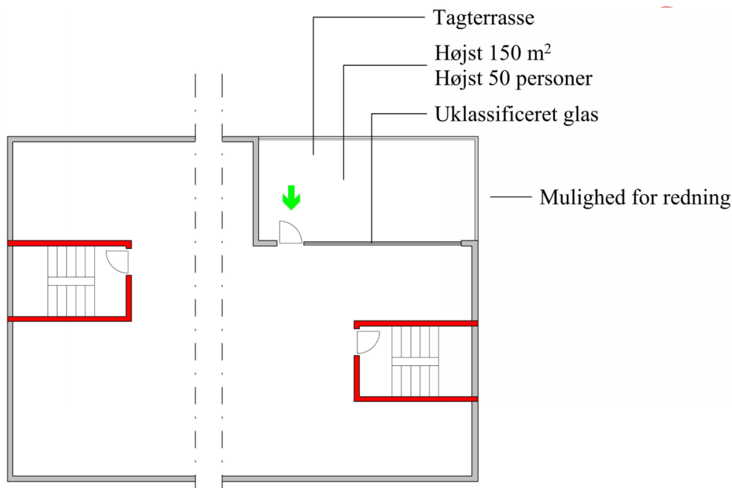
Figur 2.10. Flugtvej fra tagterrasse for bygninger, hvor gulv i øverste etage er højst 9,6 meter over terræn.
