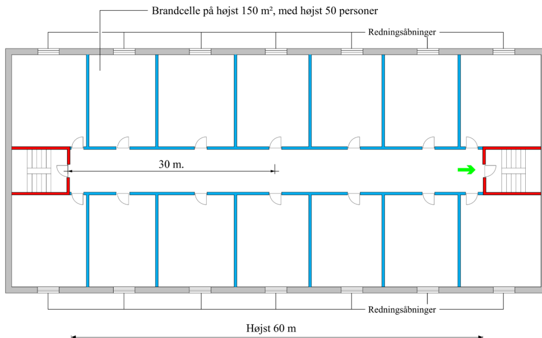
Figur 2.15. Placering af udgange fra flugtvejsgange.
