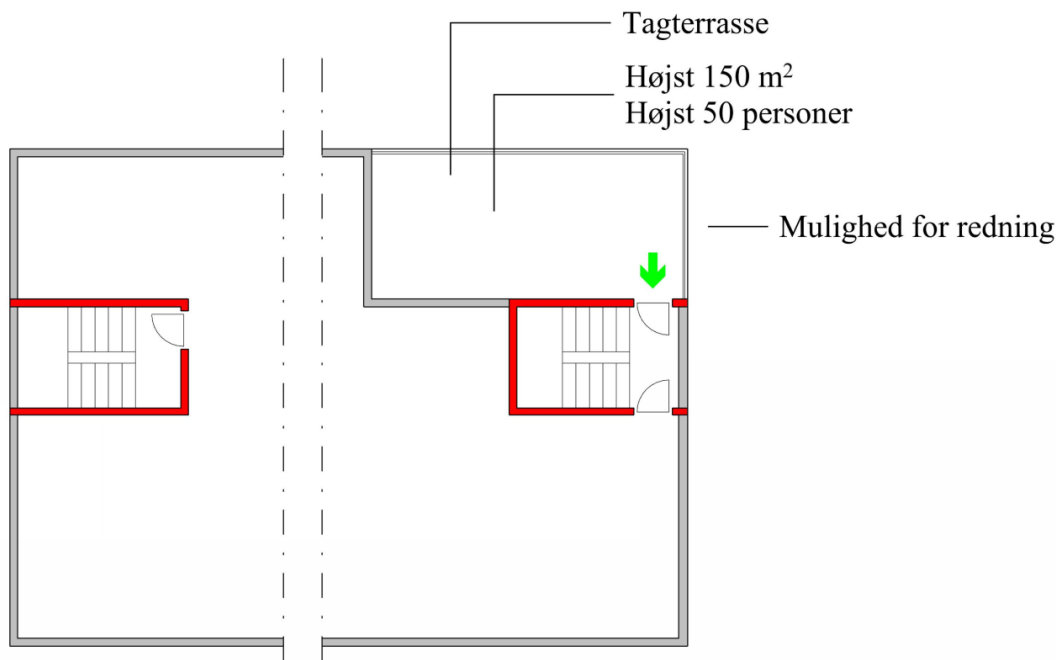
Figur 2.11. Flugtvej fra tagterrasse for bygninger, hvor gulv i øverste etage er højst 22 meter over terræn
