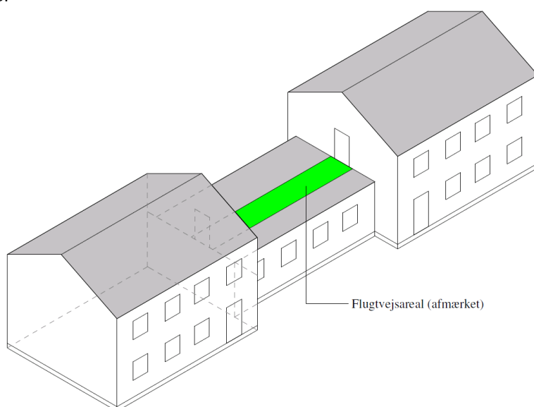
Figur Fejl! Ingen tekst med den anførte typografi i dokumentet...22. Flugtvej over tag til højst 50 personer.
