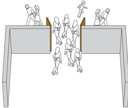
Figur Fejl! Ingen tekst med den anførte typografi i dokumentet..54 Døre fra rum til mere end 50 personer, samt fra rum på mere end 150 m 2 , til flugtvejsareal eller til det fri, skal åbne i flugtvejsretningen.
