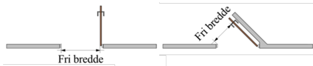
Figur 2.15. Måling af en dørs frie bredde ved henholdsvis en åbning på 90° og ved åbning på mindre end 90°.
