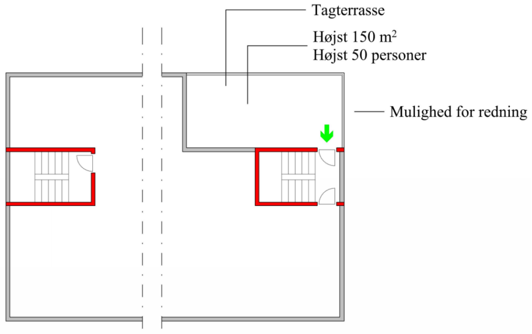
Figur 2.12. Flugtvej fra tagterrasse til trapeum for bygninger, hvor gulv i øverste etage er højst 22 meter over terræn
