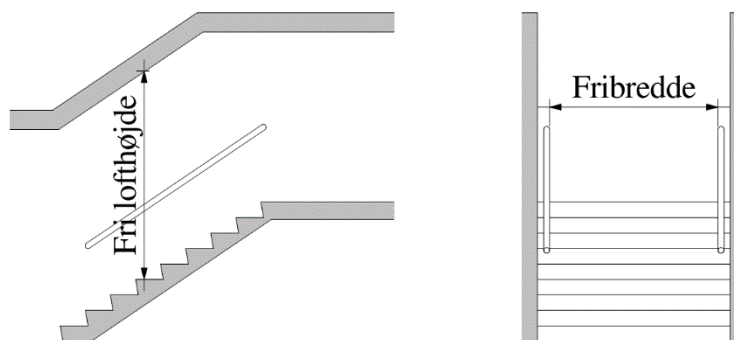
Figur 2.24. Definition af en trappes geometri.
