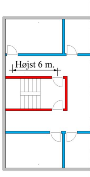
Figur 2.18. Udgang i én retning i en flugtvejsgang
