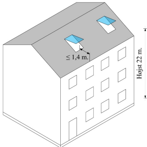
Figur 2.26. Udformning af redningsåbning i tagflade
