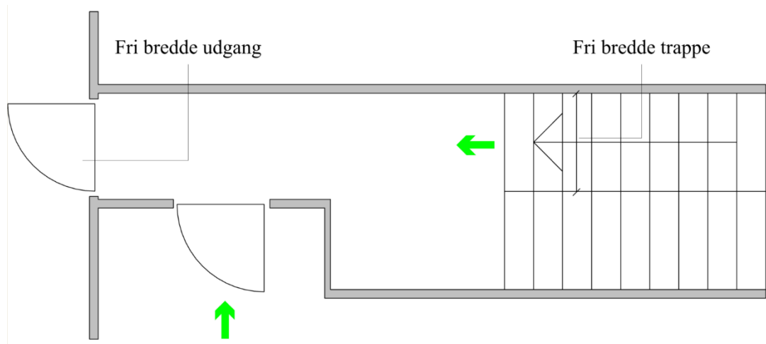
Figur 2.16. Fri bredde for udgang til det fri fra trapperum.
