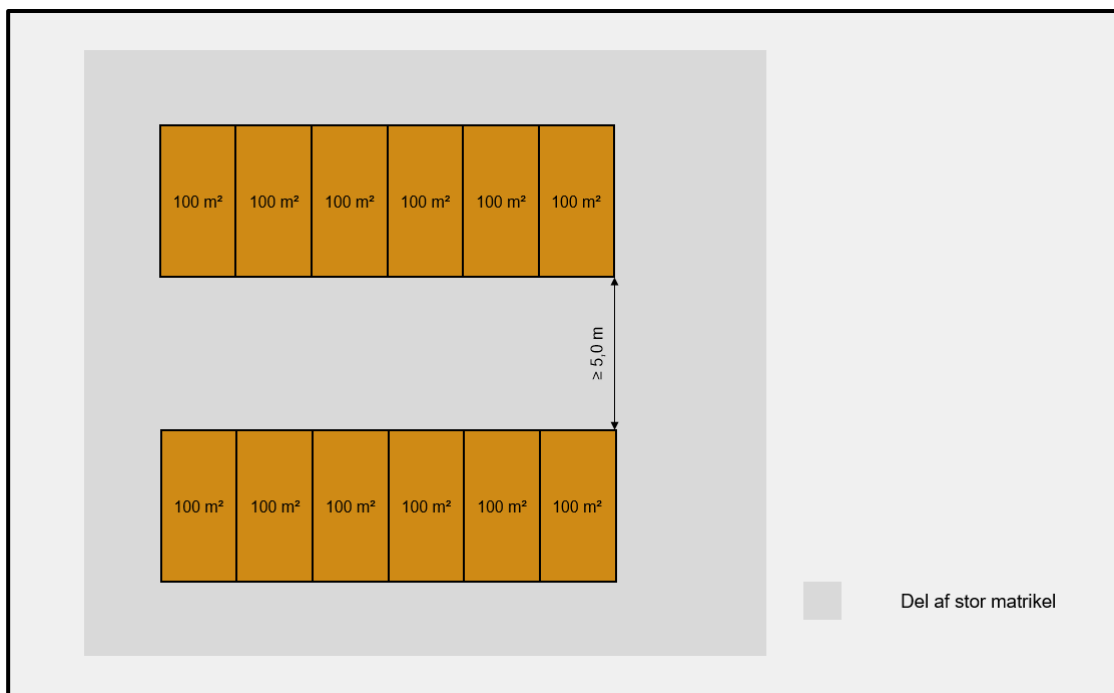
Figur 1.6.4. Rækkehusbebyggelse på højst 600 m 2 med mindst 5 m mellem de enkelte bebyggelser.
