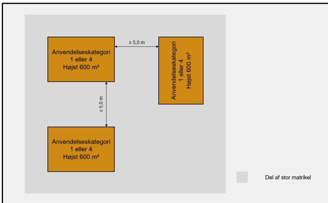
Figur 1.6.2. Brandmæssigt fritliggende bygninger i anvendelseskategori 1 eller 4.
