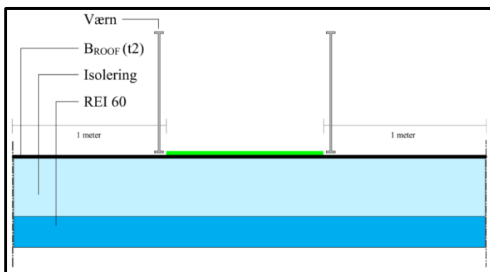
Figur 2.3.22 Brandmæssig adskillelse under flugtvej over tag. Der må ikke etableres åbninger eller gennemføringer i en afstand af min. 1 m fra kanten af flugtvejen.
