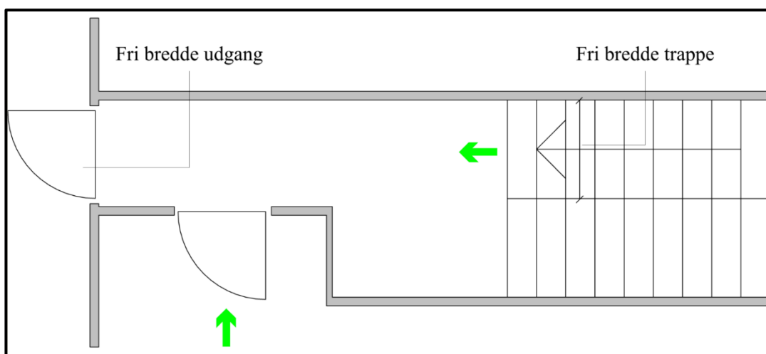
Figur 2.3.14 Fri bredde for udgang til det fri fra trapperum.
