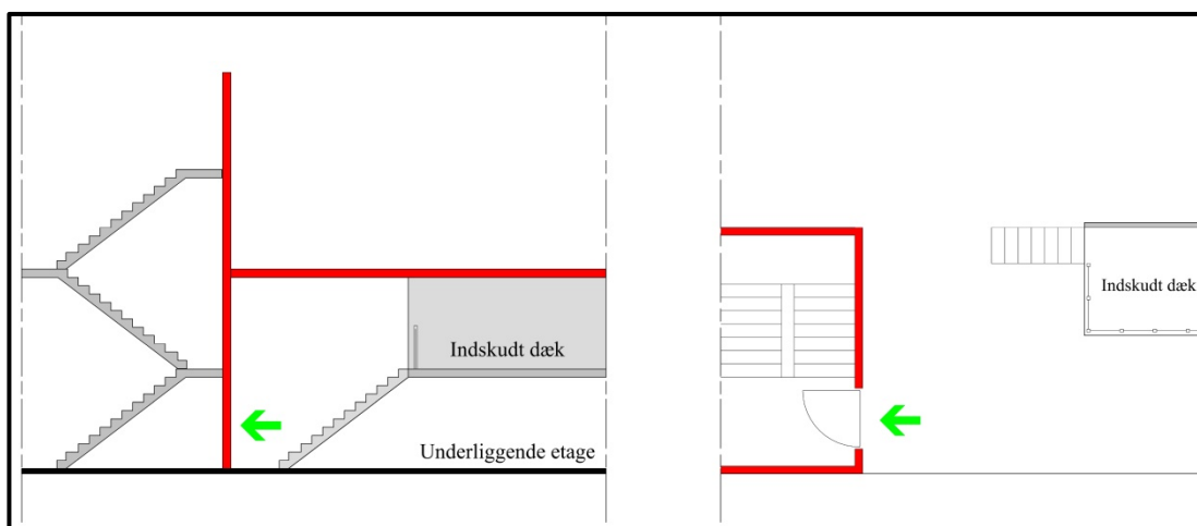
Figur 2.3.9 . Flugtvejsprincip fra en brandcelle med et indskudt dæk og hvor der ikke er adgang til flugtvejstrappe fra begge etager.
