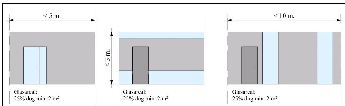
Figur 4.2.22 Præ-accepteret løsning på fordeling af gennemsigtigt glas (blå farve) uden afdækning for forskellige konfigurationer.
