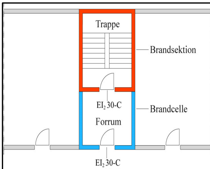
Figur 4.2.17 Præ-accepteret løsning på en trappe som er ført til kælder i en bygning, hvor gulv i øverste etage er højst 22 m over terræn.
