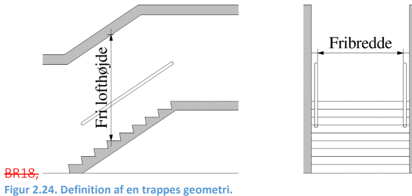
Figur 2.24. Definition af en trappes geometri.
