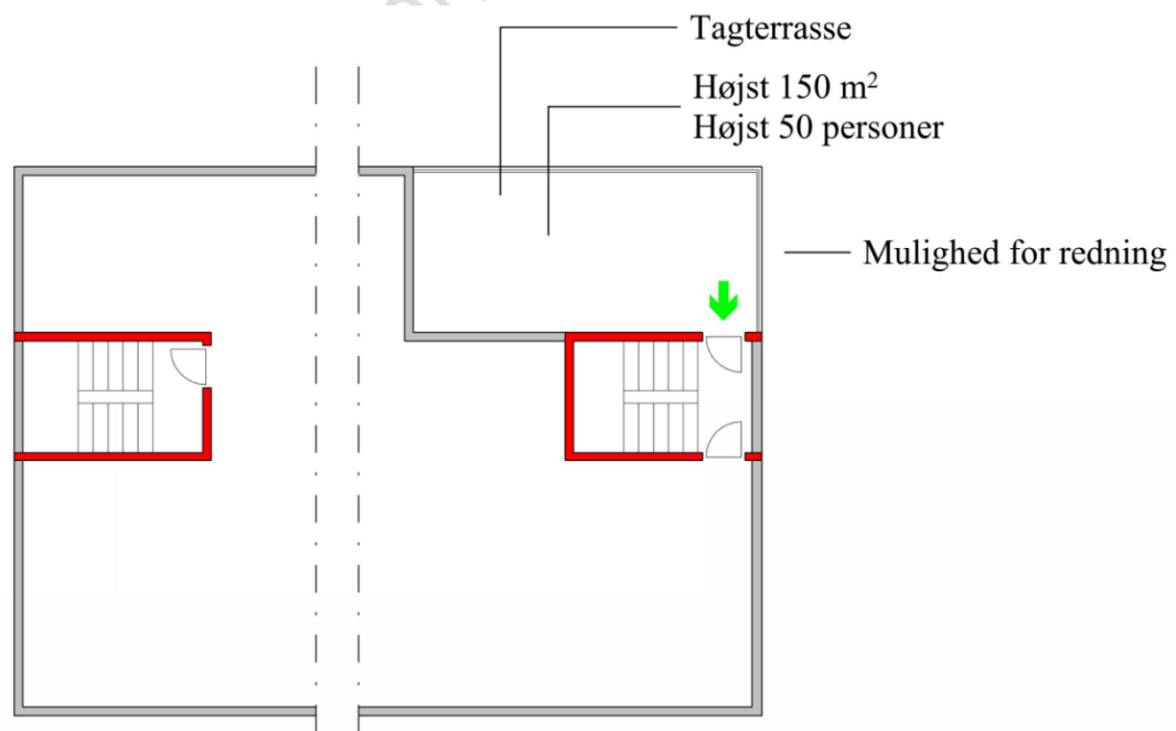
Figur 2.12. Flugtvej fra tagterrasse til trappeum for bygninger, hvor gulv i øverste etage er højst 22 meter over terræn
