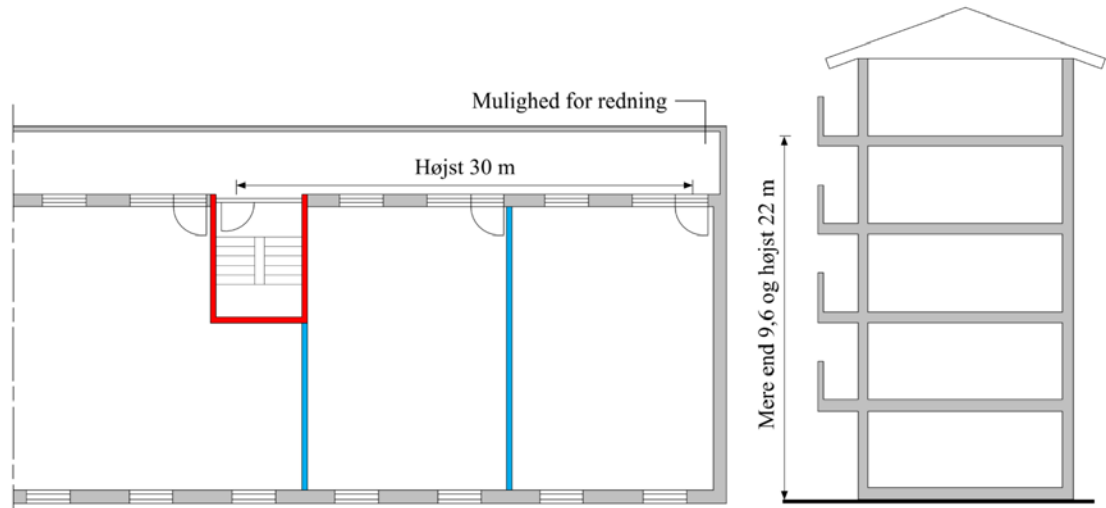
Figur 2.20. Adgang til flugtvejstrappe via altangang, hvor gulv i øverste etage er mellem 9,6 og 22 meter over terræn og redningsberedskabet kan nå enden af altangangen med deres kørbare stiger.
