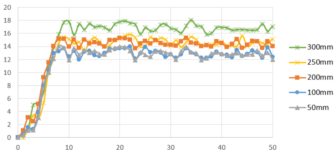
Figur 14: Eksempel på trinvis konvergens hvor resultaterne konvergerer parvist ved forøget finhed af beregningsnettet
