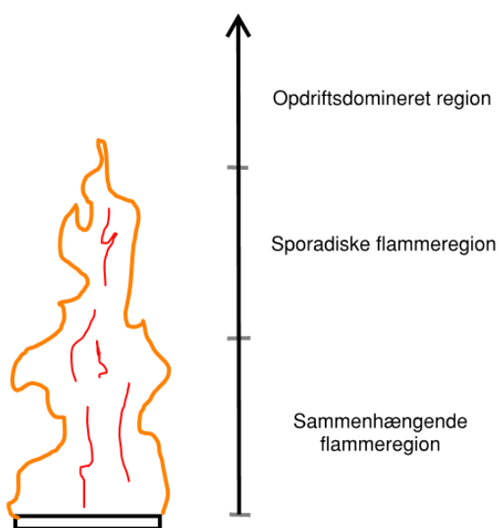
Figur 31: Regioner i McCaffrey røgfaner.
