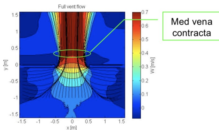
Figur 17: Modellering af blænde for strømning gennem naturlig ventilationsåbning. Lånt fra CFD Best Practice.
