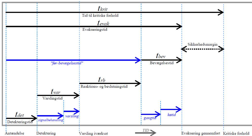
Figur 19: Evakueringstid og de enkelte tidslementer for denne, samt tiden til kritiske forhold og sikkerhedsmargin.
