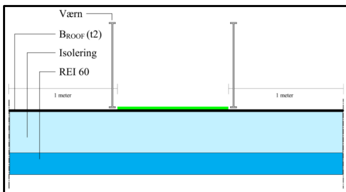
Figur 2.3.14 Brandmæssig adskillelse under flugtvej over tag. Der må ikke etableres åbninger eller gennemføringer i en afstand af min. 1 m fra kanten af flugtvejen.
