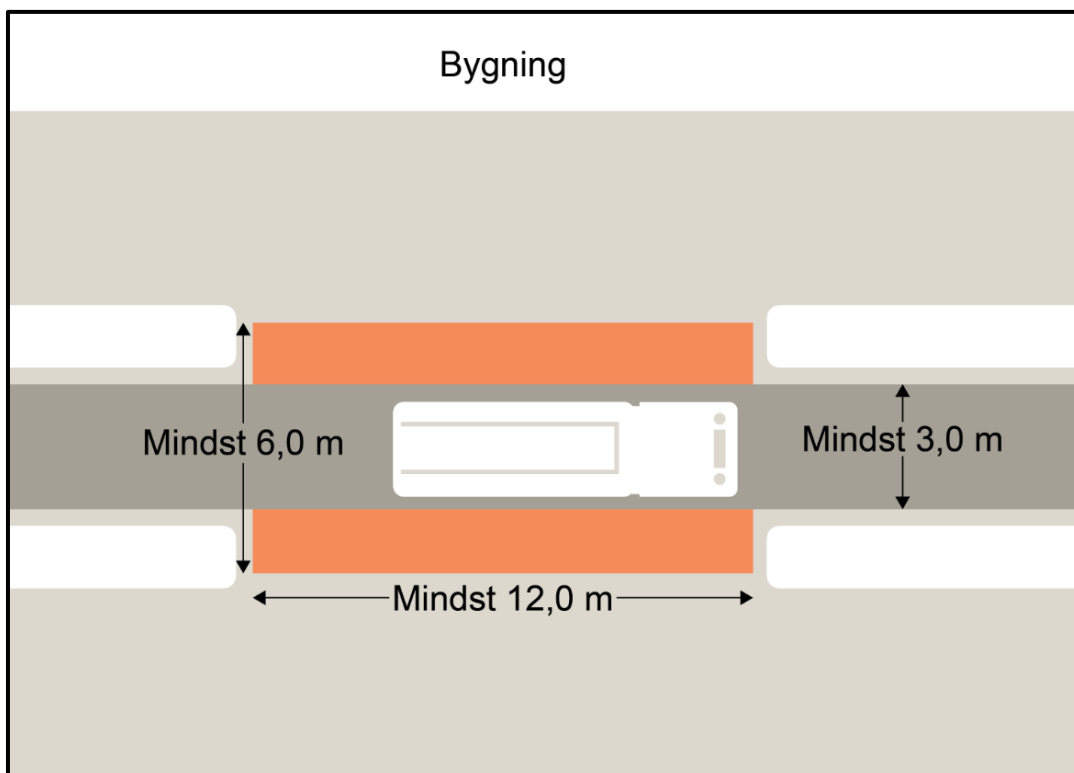
Figur 5-2 Udstigningsarealets udstrækning
