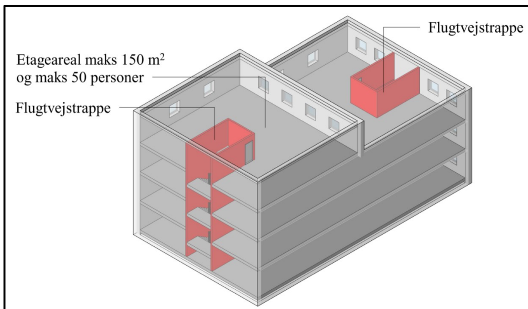
Figur 2.3.5 Brandcelle på øverste etage, hvorfra der kun er adgang til én flugtvejstrappe.
