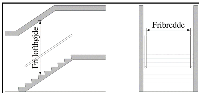
Figur 2.3.20 Definition af en trappes geometri.
