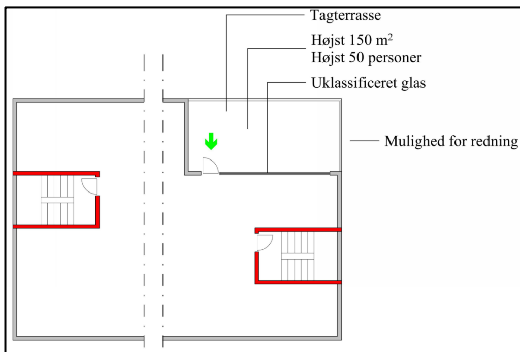
Figur 2.3.7 Flugtvej fra tagterrasse, hvor tagterrassens gulv er højst 9,6 m over terræn.
