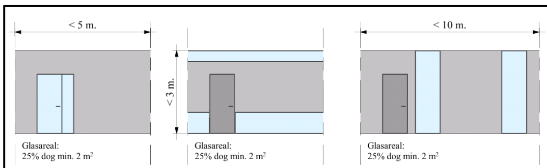
Figur 2.3.9. Præ-accepteret løsning på fordeling af gennemsigtigt glas (blå farve) uden afdækning for forskellige konfigurationer.
