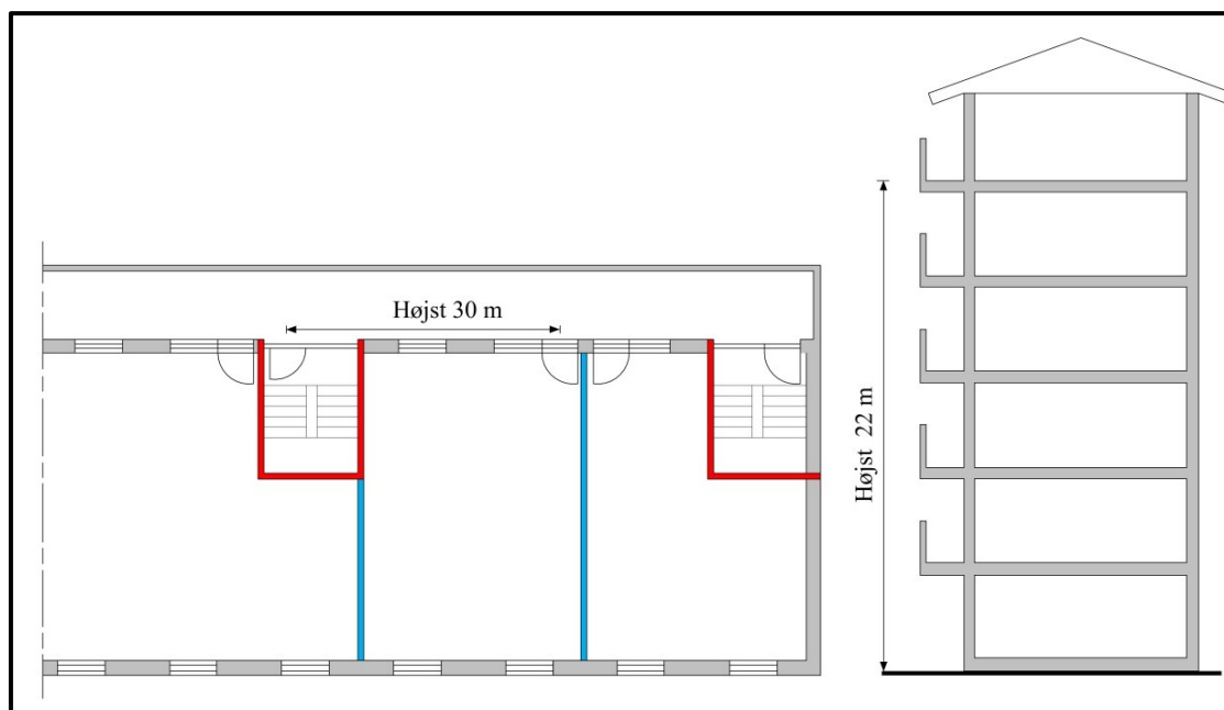
Figur 2.3.17 Adgang til flugtvejstrappe via altangang for undervisningsbygning hvor redningsberedskabet ikke kan nå altangangen med deres stiger.
