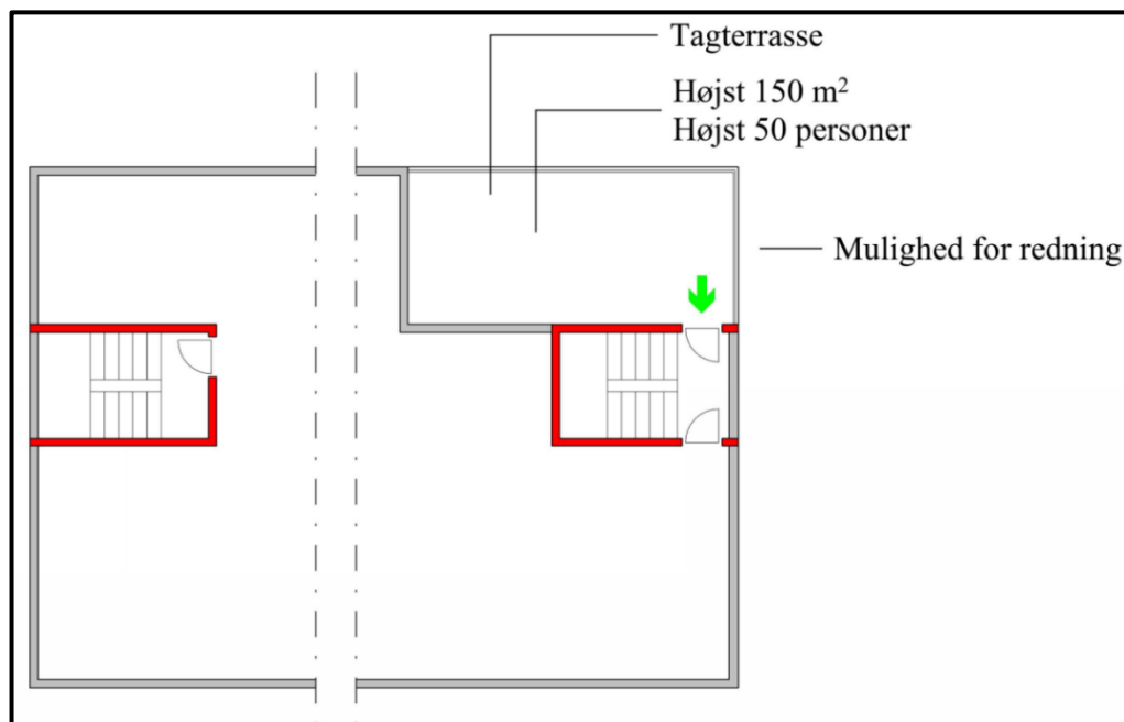
Figur 2.3.8 Flugtvej fra tagterrasse direkte til trapperum for bygninger, hvor tagterrassens gulv er højst 22 m over terræn.
