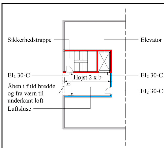
Figur 2.3.21 Princip for udførelse af luftsluse placeret over terræn for bygninger med gulv i øverste etage højst 22 m over terræn.
