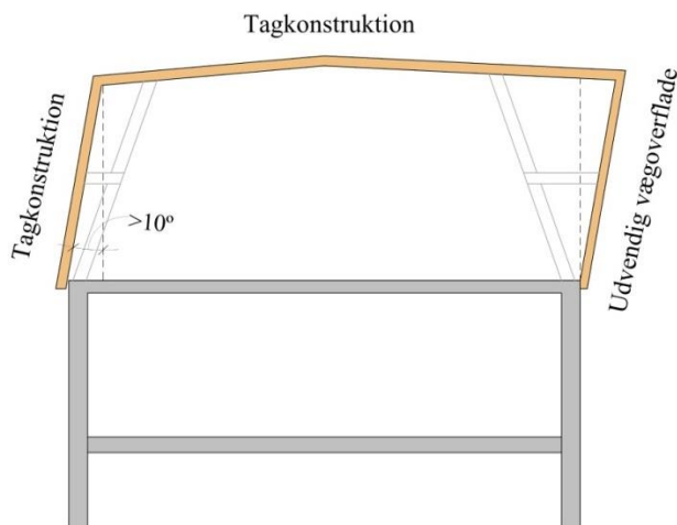
Figur 6 Definition af skrånende facade som hhv. udvendig vægoverflade og tagkonstruktion, gældende for øverste etage.
