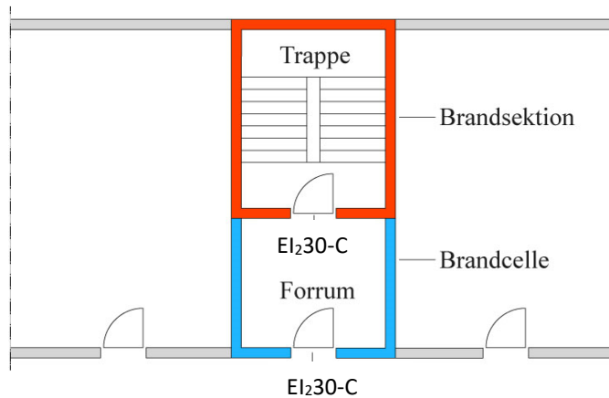
Figur 3 Trappe som er ført til kælder i en bygning, hvor gulv i øverste etage er højst 22 meter over terræn.
