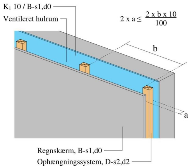
Figur 9 Beregningsmetode til den frie overflade for en regnskærms ophængningssystem.
