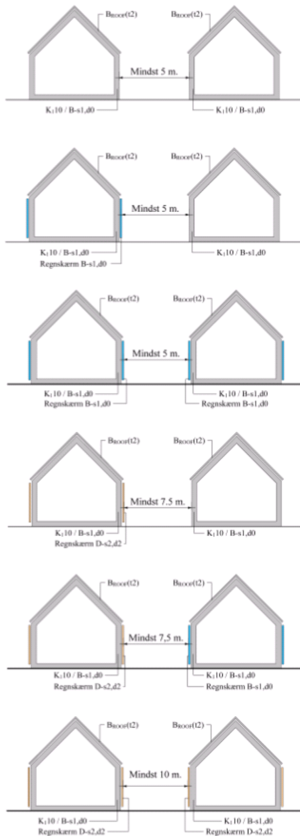
Figur 18 Afstand mellem bygninger på samme grund ift. udvendige vægoverflader.
