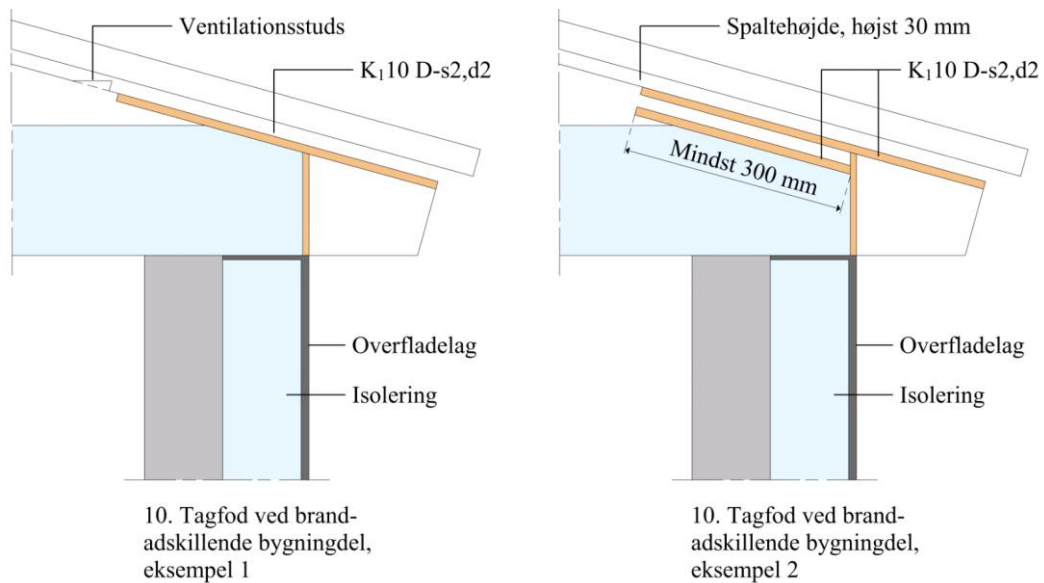
Figur 21 Ventilerede tagrum – på inddækning af isoleringsmateriale i vægge og tagkonstruktion, som ikke mindst er materiale klasse D-s2,d2 [klasse B materiale], ved tagudhæng.
