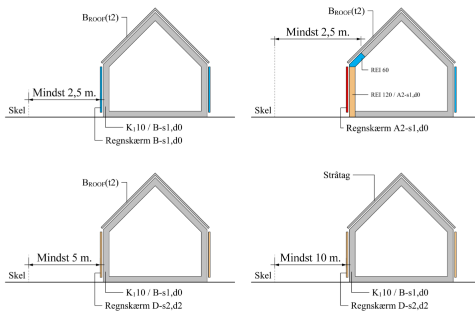
Figur 17 Afstande til skel mod nabo, vej- og stimidte fra bygningen ift. udvendige vægoverflader og tagdækning.
