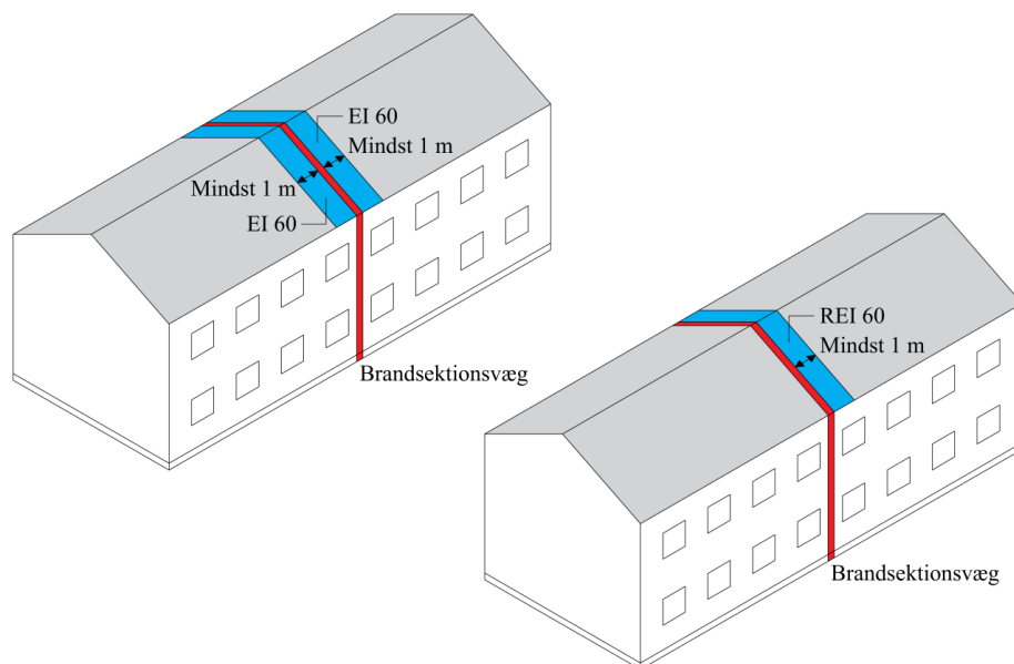
Figur 13 Brandkam og brandkamserstatning ved brandsektionsadskillelse for hindring af brandspredning over tag.
