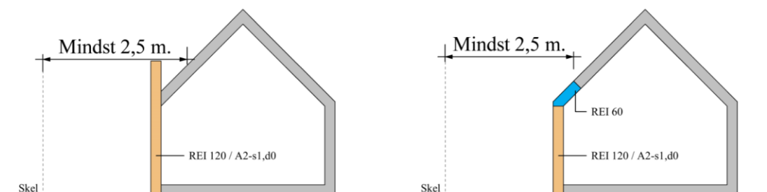
Figur 19 Brandvæg ved skel. Venstre side viser brandkam og højre side viser brandkamserstatning.
