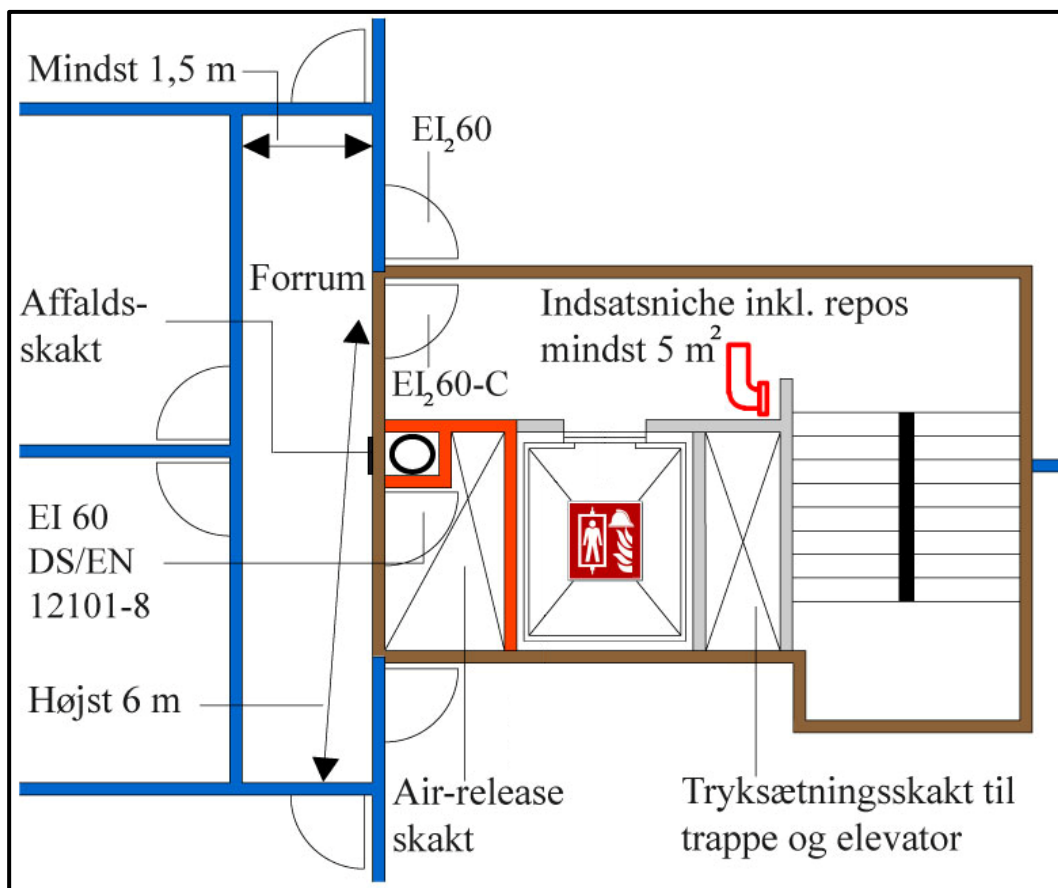
Figur 5.4.3.2.b: Eksempel nr. 02 for tryksat trapperum.
