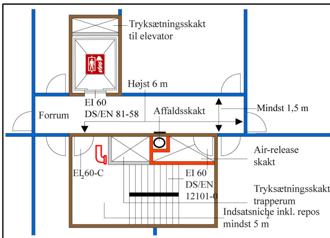
Figur 5.4.3.2.c: Eksempel nr. 03 for tryksat trapperum.
