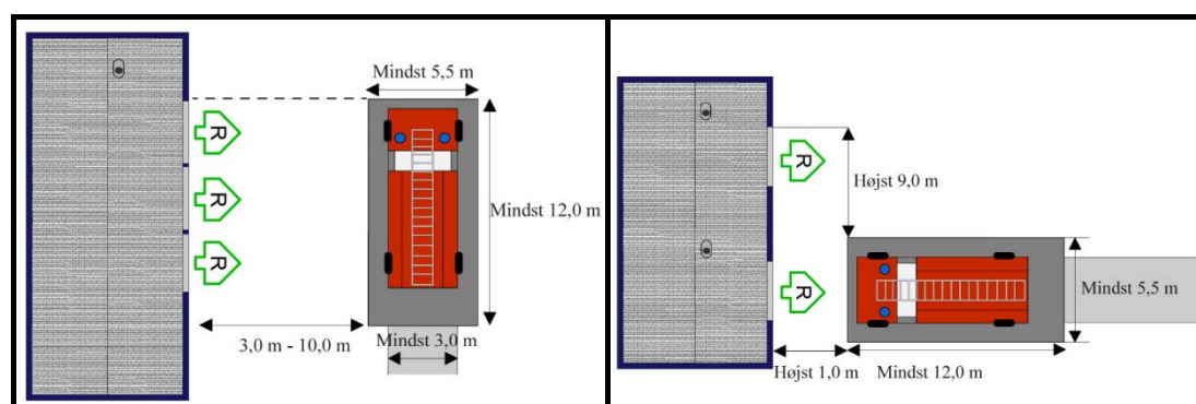
Figur 5.2.3.2.b: Afstand til bygning for kørbare stiger.
