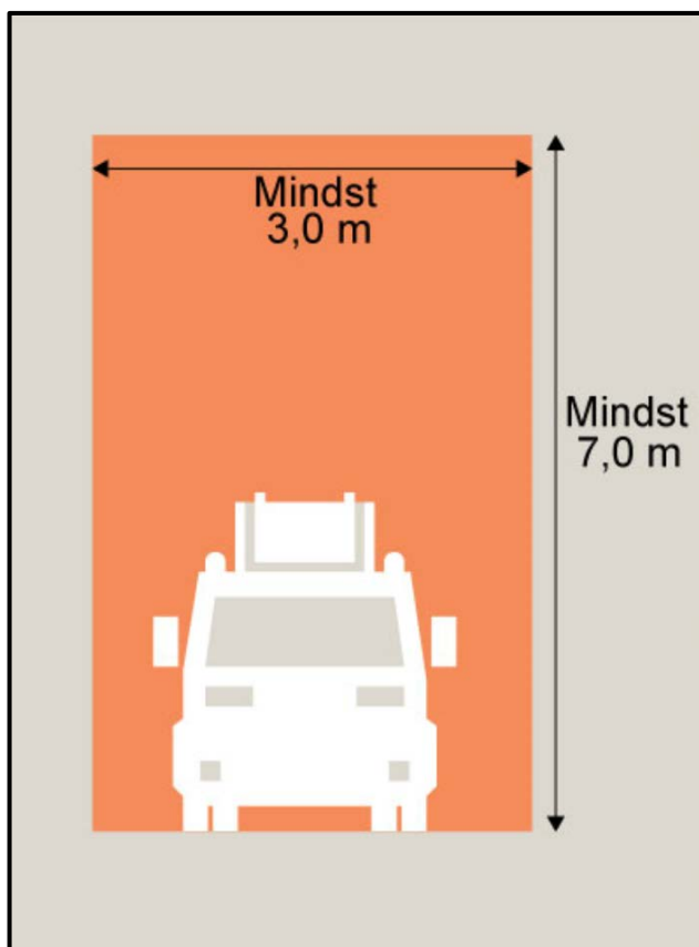
Figur 5.2.4.a: Frihøjde over brandvej ved udstigningsarealer.
