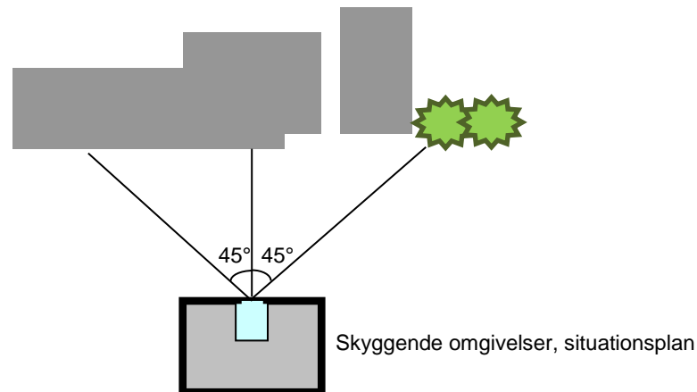
Figur 2. Illustration af skyggende omgivelser. Korrektionsfaktoren er bestemt af middelværdien af profilvinklen for skyggegeverne, som befinder sig inden for en vinkel på \pm 45^\circ i forhold til et lodret plan gennem midten af vinduet.
