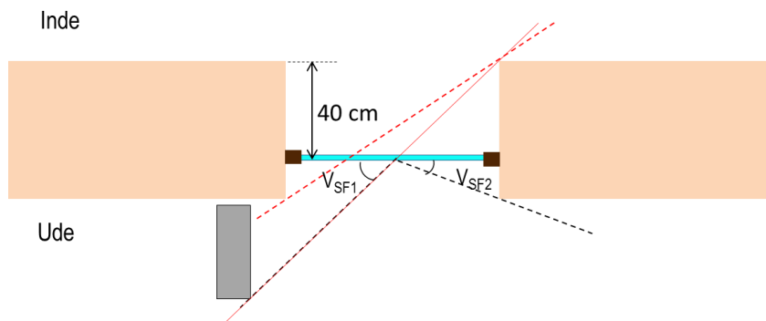
Figur 9. Vandret snit, der illustrerer at skygeeffekterne fra den tykke vinduesvæg og fra fremspringet ved siden af vinduet overlapper. Den resulterende skyggeeffekt kan beregnes som produktet af korrektionsfaktorerne for de to forskellige fremspring ved siden af vinduet og fremspringet over vinduet.
