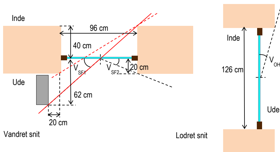
Figur 10. Skitser til bestemmelse af korrektionsfaktorer for vinduet beskrevet i eksemplet.
