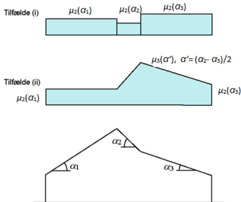
Figur F.3 NA - Formfaktorer for tagflade med ændring i hældning
