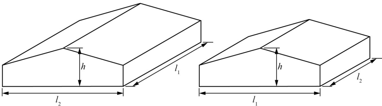
Figur 5.0.b NA – Dimensioner på bygning
