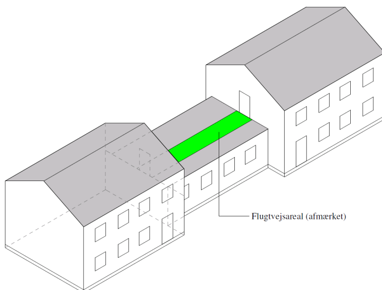
Figur Fejl! Ingen tekst med den anførte typografi i dokumentet...22. Flugtvej over tag til højst 50 personer.
