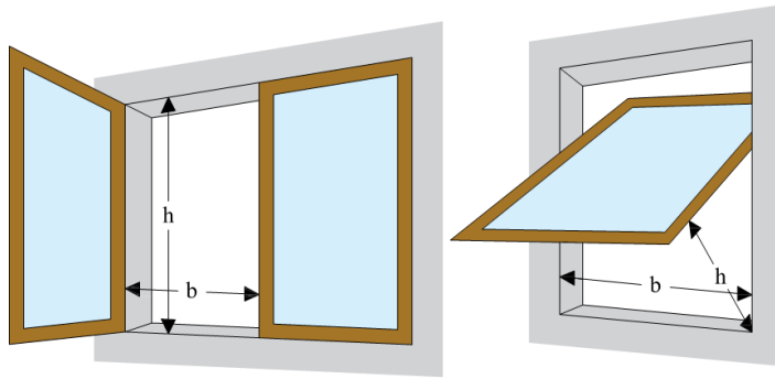
Figur Fejl! Ingen tekst med den anførte typografi i dokumentet..105. Udformning af redningsåbning til personredning.
