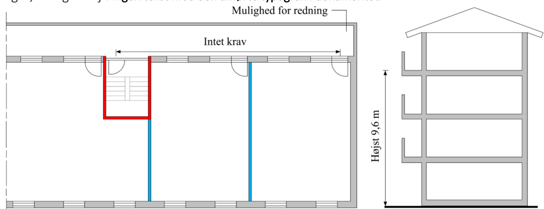
Figur Fejl! Ingen tekst med den anførte typografi i dokumentet..19. Adgang til flugtvejstrappe via altangang, hvor gulv i øverste etage er højst 9,6 meter over terræn og redningsberedskabet kan nå altangangen med deres bærbare stiger.
