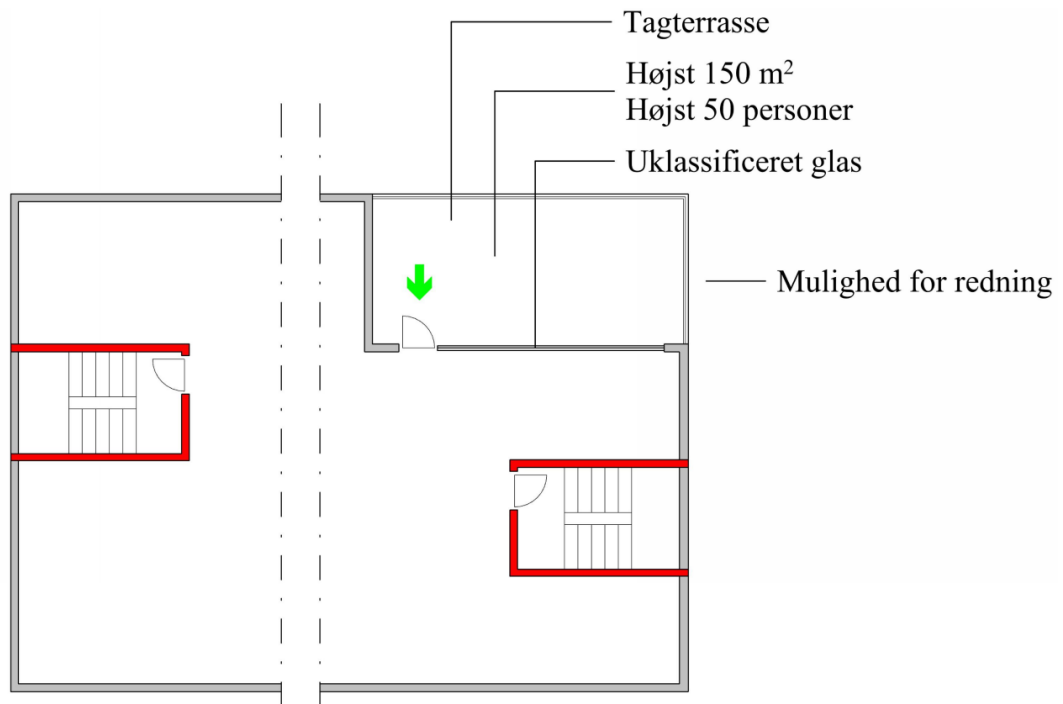
Figur Fejl! Ingen tekst med den anførte typografi i dokumentet..11. Flugtvej fra tagterrasse for bygninger, hvor gulv i øverste etage er højst 9,6 meter over terræn.
