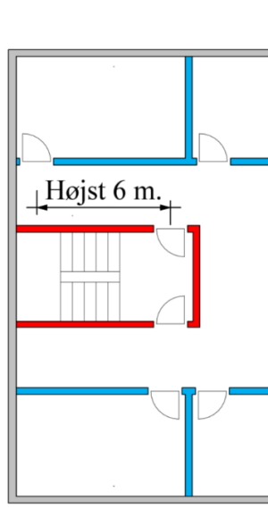
Figur Fejl! Ingen tekst med den anførte typografi i dokumentet..98. Udgang i én retning i en flugtvejsgang
