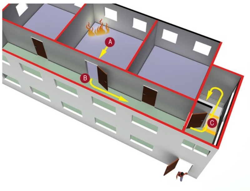
Figur Fejl! Ingen tekst med den anførte typografi i dokumentet..1. Princip for evakuering til terræn i det
