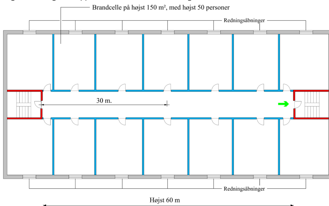
Figur Fejl! Ingen tekst med den anførte typografi i dokumentet..87. Placering af udgange fra flugtvejsgange.
