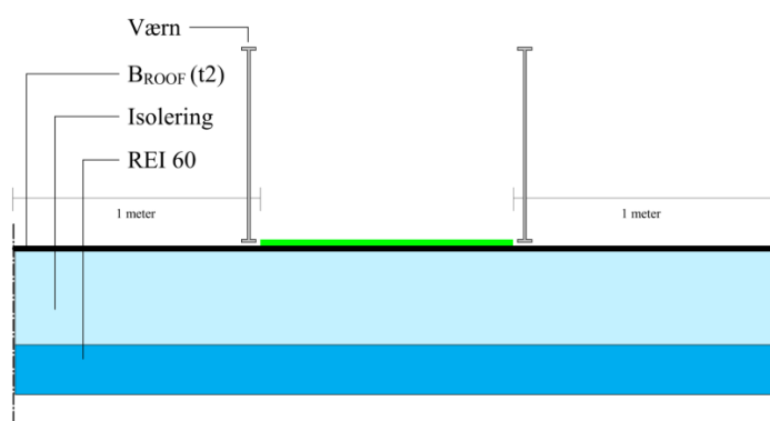
Figur Fejl! Ingen tekst med den anførte typografi i dokumentet...23. Brandmæssig adskillelse under flugtvej over tag. Der må ikke etableres åbninger eller gennemføringer i en afstand af min. 1 meter fra kanten af flugtvejen.
