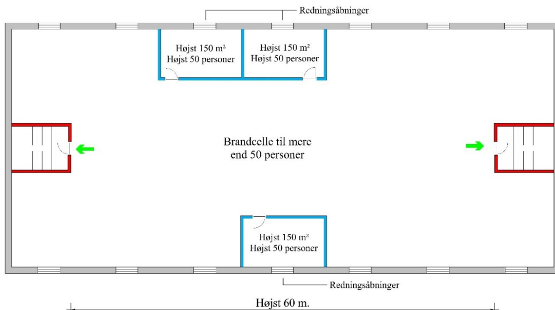
Figur Fejl! Ingen tekst med den anførte typografi i dokumentet..6. Udgang fra en indeliggende brandcelle via en anden brandcelle.
