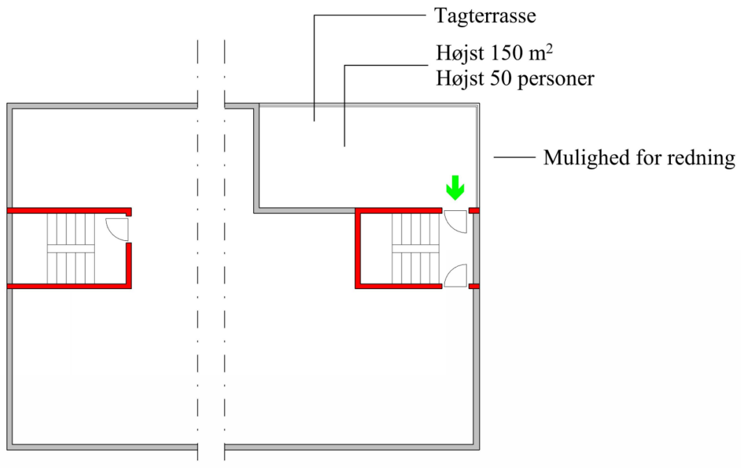
Figur Fejl! Ingen tekst med den anførte typografi i dokumentet..12. Flugtvej fra tagterrasse for bygninger, hvor gulv i øverste etage er højst 22 meter over terræn
