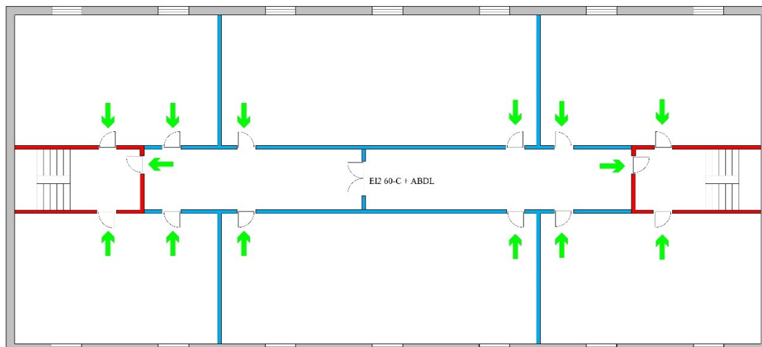
Figur Fejl! Ingen tekst med den anførte typografi i dokumentet..10. Opdeling af flugtvejsgang for etablering af uafhængige flugtveje fra opholdsrum.
