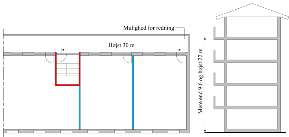
Figur Fejl! Ingen tekst med den anførte typografi i dokumentet..20. Adgang til flugtvejstrappe via altangang, hvor gulv i øverste etage er mellem 9,6 og 22 meter over terræn og redningsberedskabet kan nå enden af altangangen med deres kørbare stiger.
