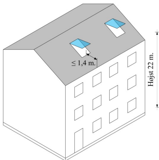
Figur Fejl! Ingen tekst med den anførte typografi i dokumentet..116. Udformning af redningsåbning i tagflade
