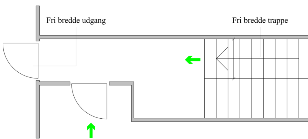
Figur Fejl! Ingen tekst med den anførte typografi i dokumentet..76. Fri bredde for udgang til det fri fra trapperum.
