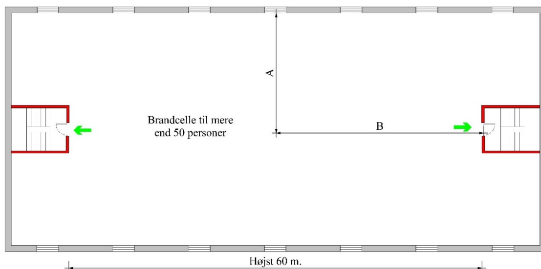
Figur Fejl! Ingen tekst med den anførte typografi i dokumentet..9. Døre til flugtveje fra brandcelle med mere end 50 personer, men mindre end 150 personer.
