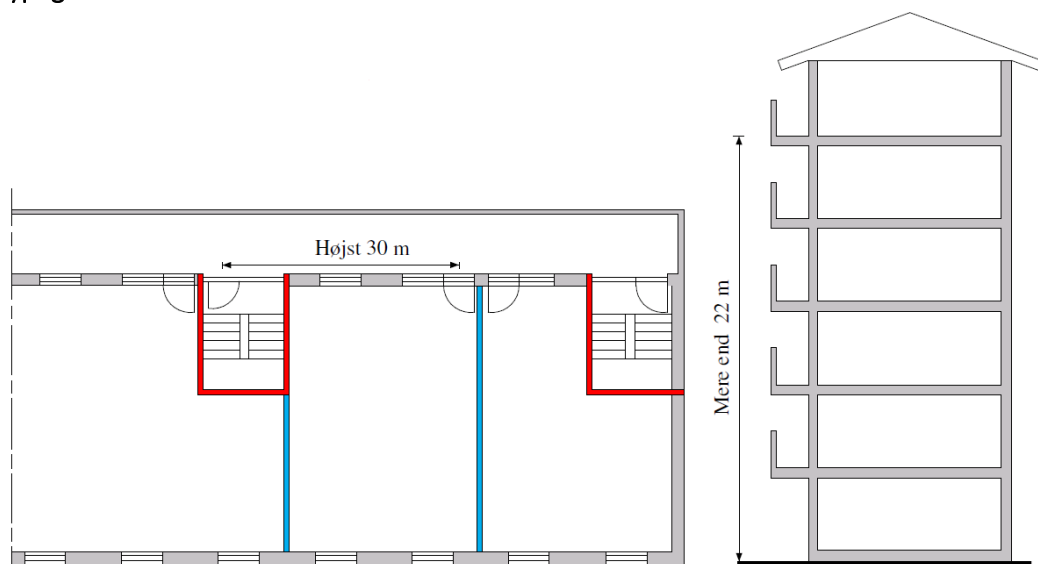
Figur Fejl! Ingen tekst med den anførte typografi i dokumentet..21. Adgang til flugtvejstrappe via altangang, hvor gulv i øverste etage er mere end 22 meter over terræn eller hvor redningsberedskabet ikke kan nå altangangen med deres stiger.
