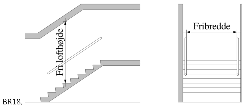
Figur Fejl! Ingen tekst med den anførte typografi i dokumentet..24. Definition af en trappes geometri.
