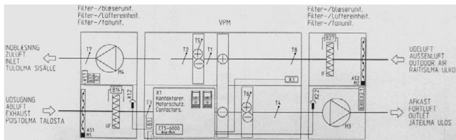
Figur 23. Anlægsdiagram. (Nilan A/S)
