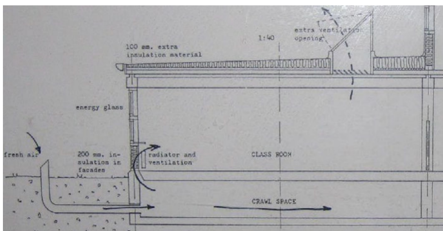
Figur 57. Principsnit. (Skolen)
