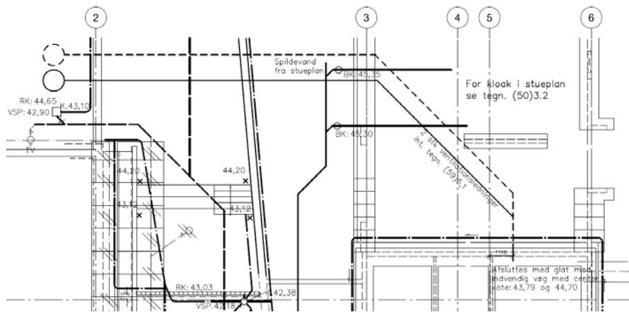
Figur 22. Udsnit af kloakplan, se figur 21.
