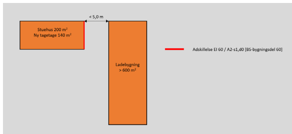
Figur 1.6. Flere bygninger i anvendelseskategori 1 eller 4, hvor der mellem bygningerne er mindst 5,0 m.
