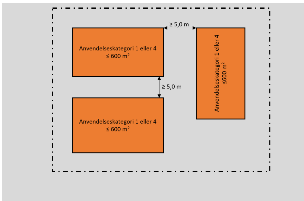
Figur 1.2. Flere bygninger med afstand imellem i anvendelseskategori 1 eller 4.
