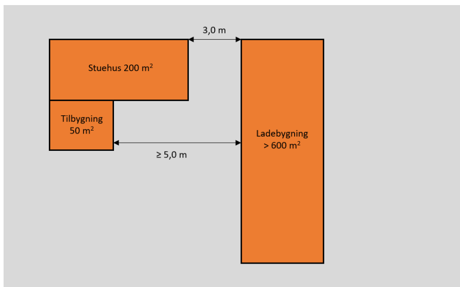
Figur 1.5. Tilbygning til eksisterende stuehus, hvor tilbygningen er fritliggende i forhold til en eksisterende ladebygning.
