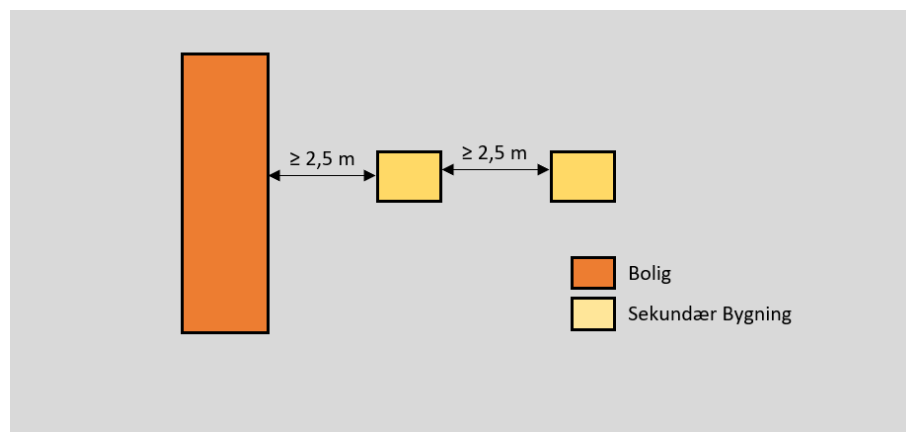
Figur 1.10. Placering af flere fritliggende sekundære bebyggelser.
