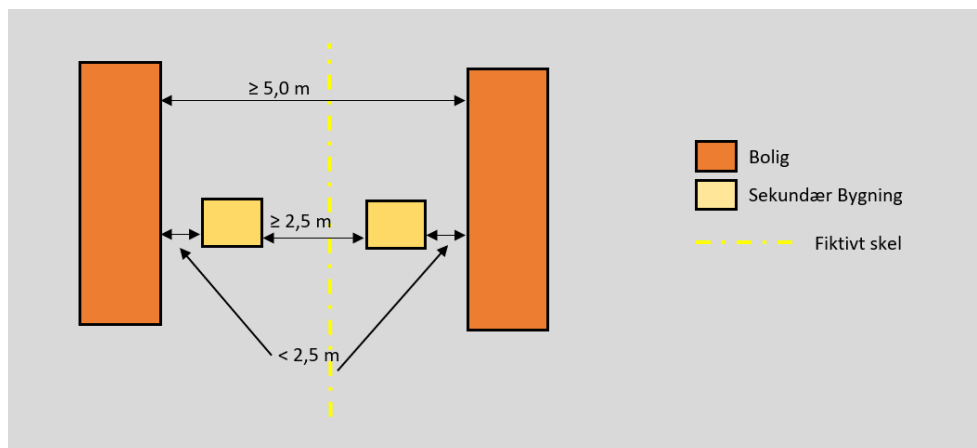
Figur 1.8. Placering af sekundær i forhold til primær bebyggelse på en stor grund.
