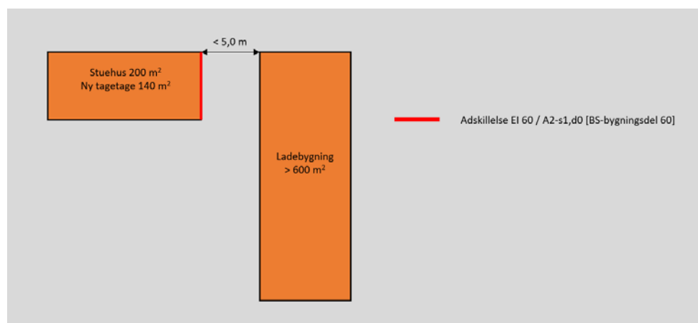
Figur 1.6. Flere bygninger i anvendelseskategori 1 eller 4, hvor der mellem bygningerne er mindst 5,0 m.
