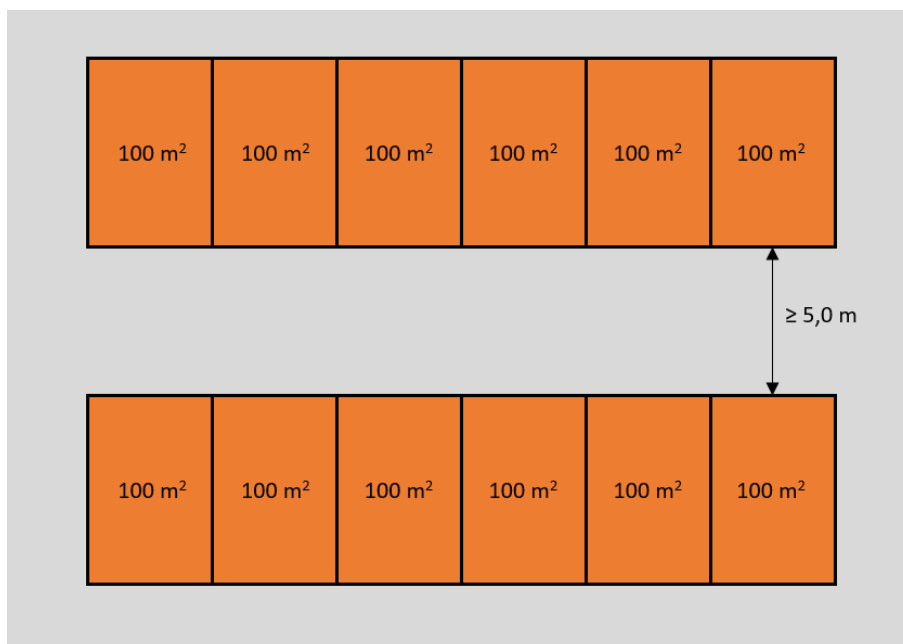
Figur 1.4. Rækkehusbebyggelse på op til 600 \text{ m}^2 med mindst 5 \text{ m} mellem de enkelte bebyggelser.
