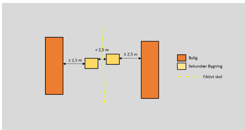
Figur 1.9. Placering af sekundær i forhold til primær bebyggelse på en stor grund.
