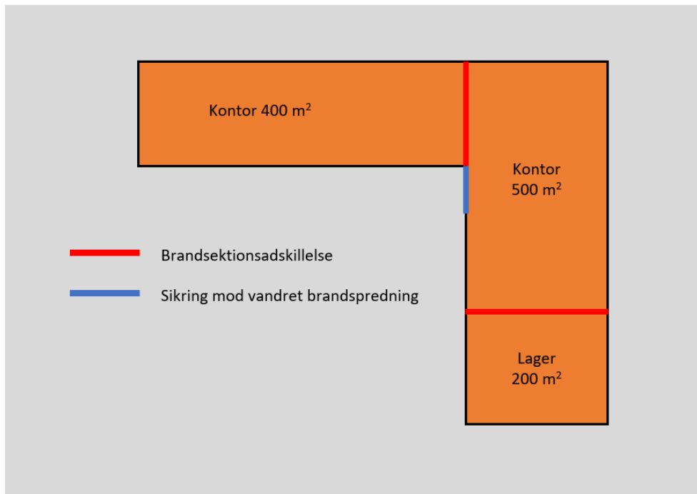
Figur 1.3. En bygning større end 600 m 2 opdelt med brandsektionsadskillelse.
