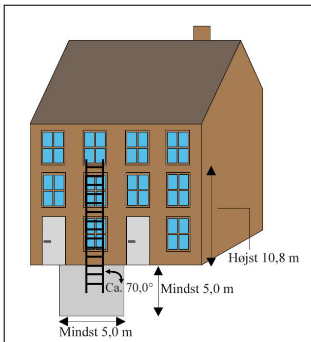
Figur 5.2.3.3.a: Opstilling af bærbare stige
