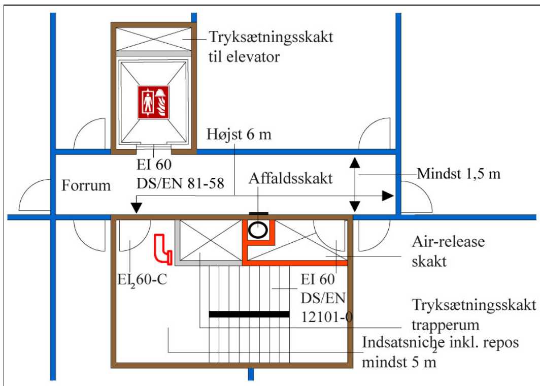
Figur 5.4.3.2.b: Eksempel nr. 02 for tryksat trapperum
