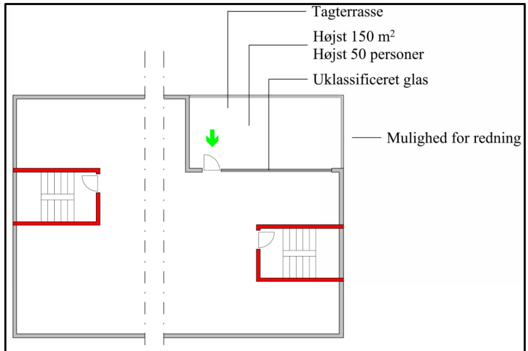
Figur 2.3.10 Flugtvej fra tagterrasse, hvor tagterrassens gulv er højest 9,6 m over terræn.
