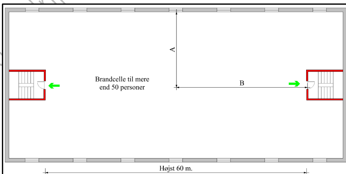
Figur 2.3.7 Døre til flugveje fra brandcelle med flere end 50 personer, men færre end 150 personer.
