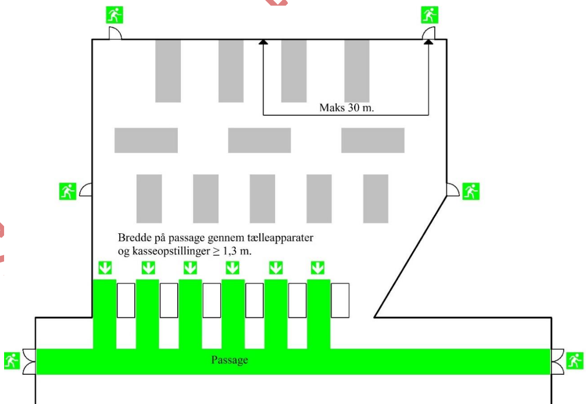
Figur 2.9. Præ-accepteret løsning for flugtveje fra butik med kasseopstilling. Passage (grøn markering) udføres med en fri bredde på minimum 1,3 meter. Primære flugtvejsdøre skal minimum være 1,2 m i fri bredde.
