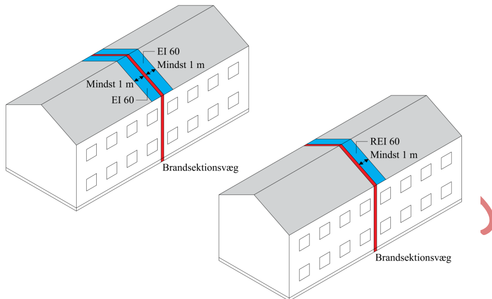
Figur 4.14. Brandkam og brandkammerstatning ved brandsektionsadskillelse for hindring af brandspredning over tag.
