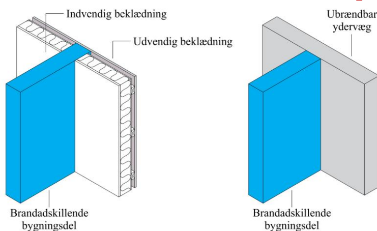
Figur 4.11 Sammenbygning af facade og brandadskillelende bygningsdel, hvor den brandadskillelende væg føres frem til indersiden af den udvendige beklædning. Samme princip gælder for etageadskillelser.
