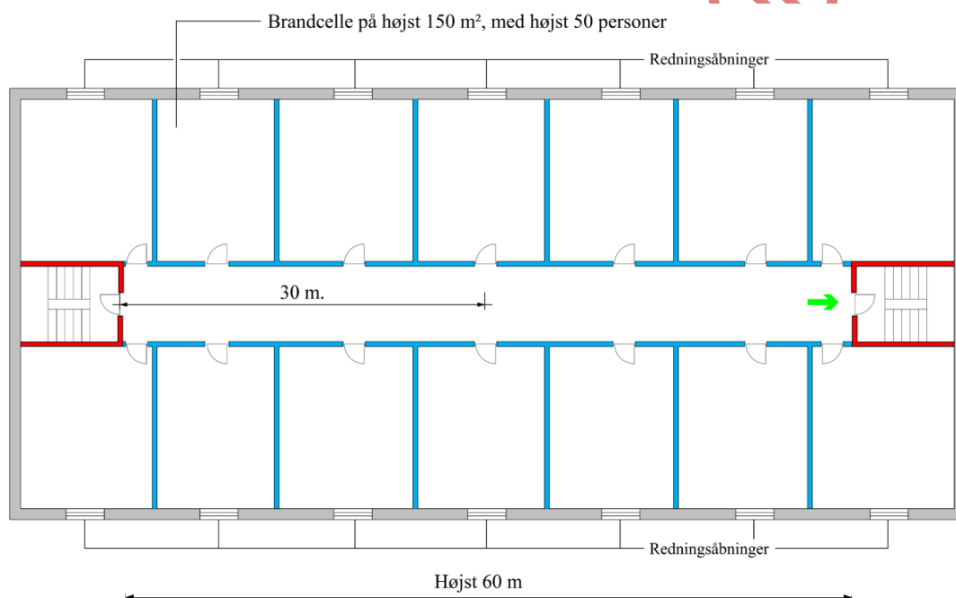
Figur 2.16. Placering af udgange fra flugtvejsgange.
