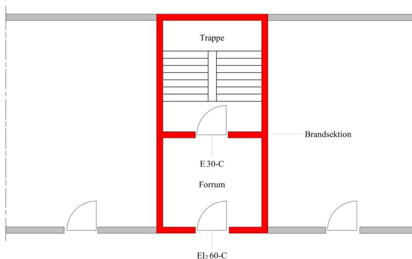
Figur 4.17. Præ-accepteret løsninger på en trappe som er ført til kælder i en bygning med forsamlingslokaler, butikker mv., hvor gulv i øverste etage er højst 22 meter over terræn.
