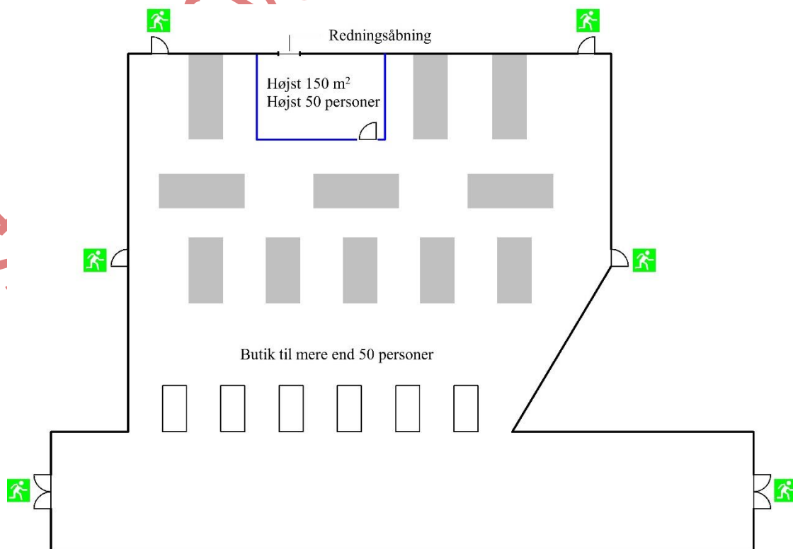
Figur 2.5. Udgang fra en indeliggende brandcelle via en anden brandcelle.
