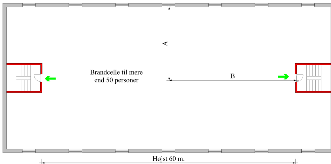
Figur 2.6. Døre til flugtveje fra brandcelle med mere end 50 personer, men mindre end 150 personer.
