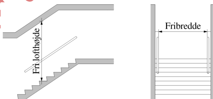
Figur 2.23. Definition af en trappes geometri.
