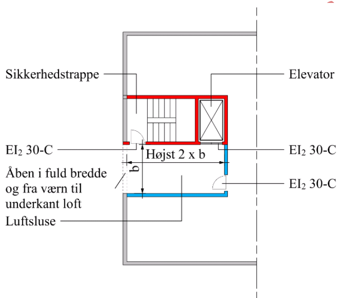
Figur 2.24. Princip for udførelse af luftsluse placeret over terræn for bygninger med gulv i øverste etage højst 22 meter over terræn.
