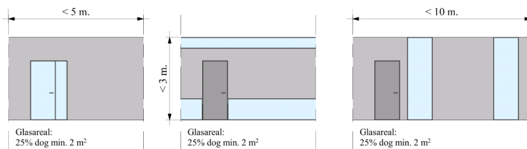
Figur 2.12. Præ-accepteret løsning på fordeling af gennemsigtigt glas (blå farve) uden afdækning for forskellige konfigurationer.
