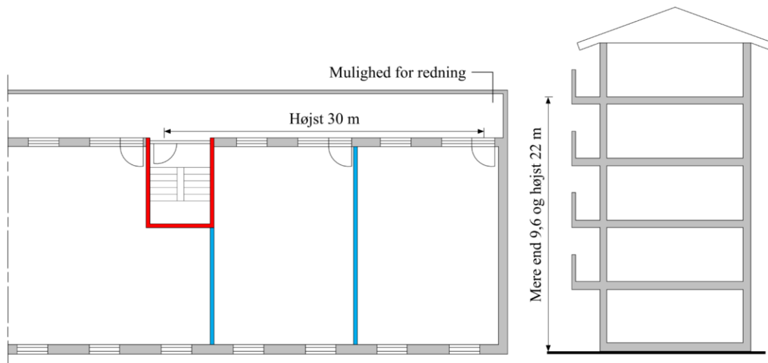
Figur 2.19. Adgang til flugtvejstrappe via altangang for bygning med forsamlingslokaler, butikker mv., hvor gulv i øverste etage er mellem 9,6 og 22 meter over terrænen og redningsberedskabet kan nå enden af altangangen med deres kørbare stiger.
