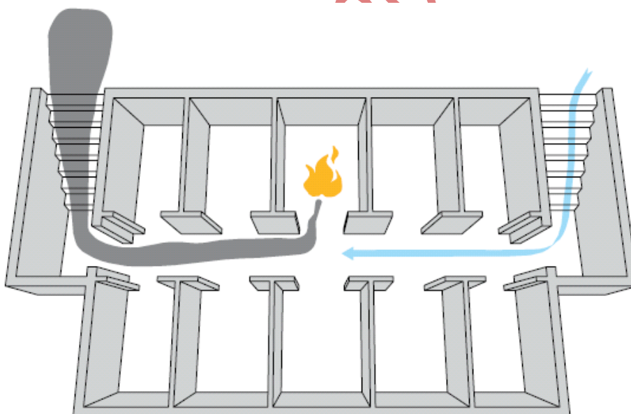
Figur 5.3 Præ-accepteret løsning på røgudluftning af kældre.
