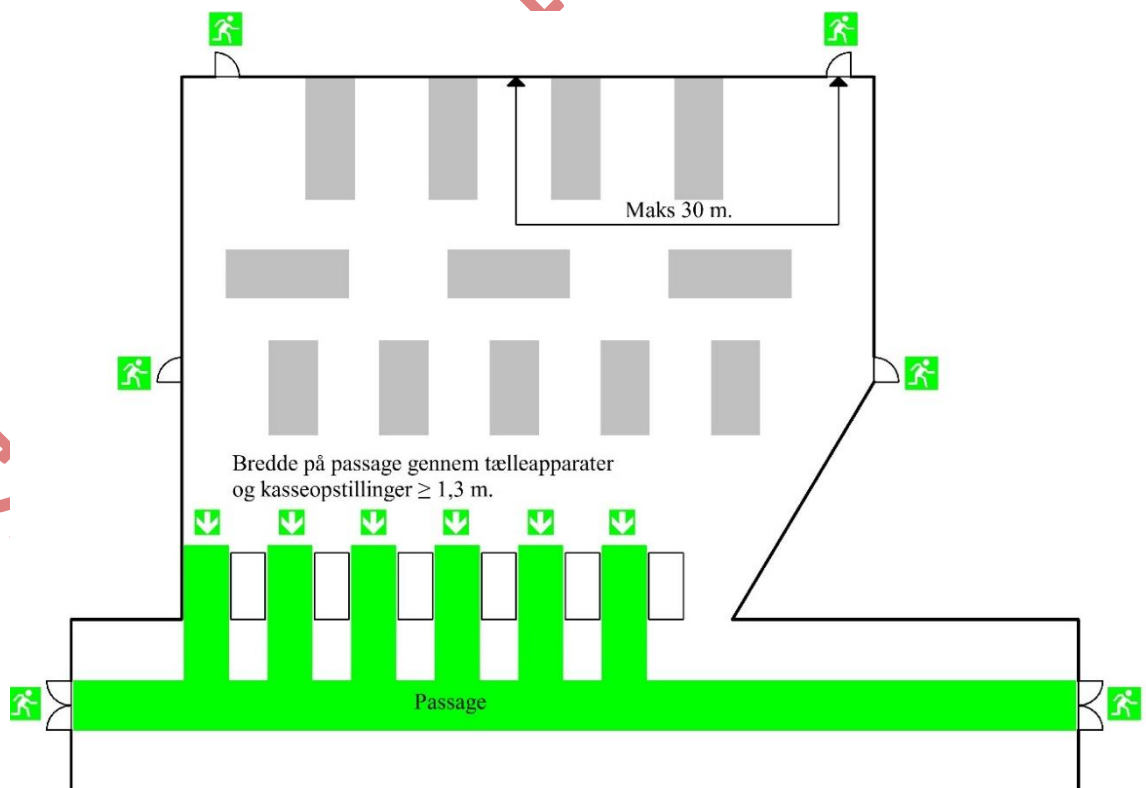
Figur 2.9. Præ-accepteret løsning for flugtveje fra butik med kasseopstilling. Passager (grøn markering) udføres med en fri bredde på minimum 1,3 meter. Primære flugtvejsdøre skal minimum være 1,2 m i fri bredde.
