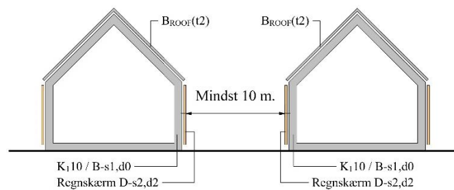
Figur 4.2 Afstand mellem bygninger på samme grund ift. udvendige vægoverflader. Alle klassifikationer er minimumskrav.
