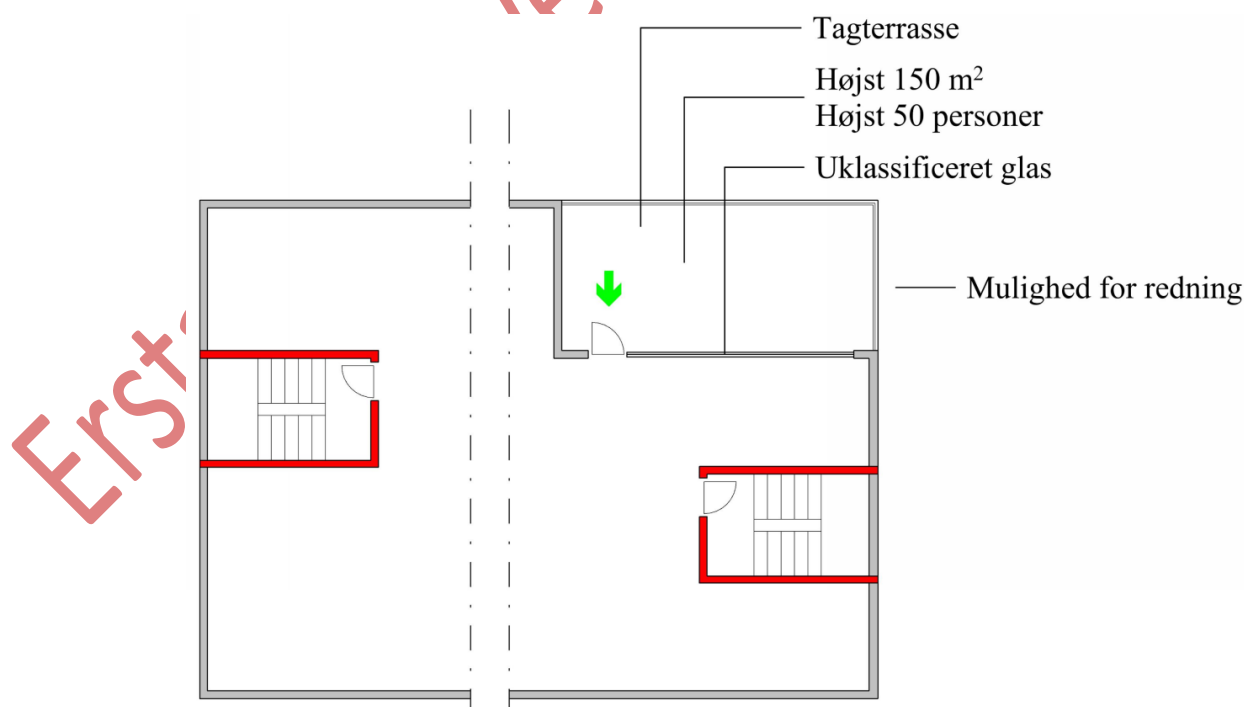
Figur 2.10. Flugtvej fra tagterrasse for bygninger, hvor gulv i øverste etage er højst 9,6 meter over terræn.
