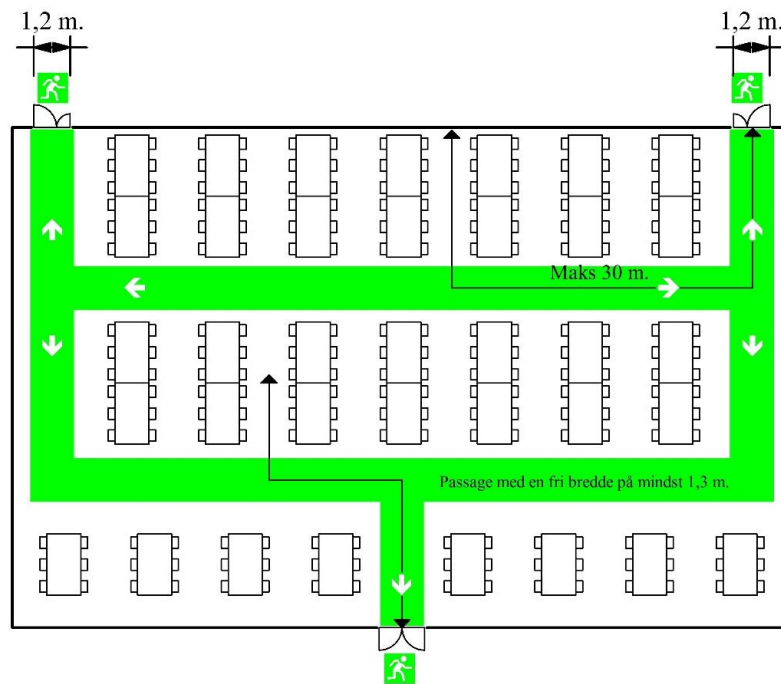
Figur 2.8. Præ-accepteret løsning for forsamlingslokale med passager på minimum 1,3 meter fri bredde.
