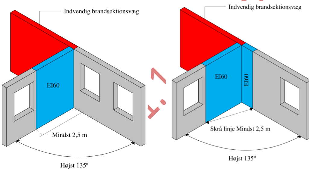
Figur 4.12 (fortsat) Sikring af vandret brandspredning/vinkelsmitte ved brandsektionsafgrænsende vægge.
