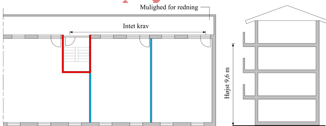
Figur 2.18. Adgang til flugtvejstrappe via altangang for bygning med forsamlingslokaler, butikker mv., hvor gulv i øverste etage er højst 9,6 meter over terræn og redningsberedskabet kan nå altangangen med deres bærbare stiger.
