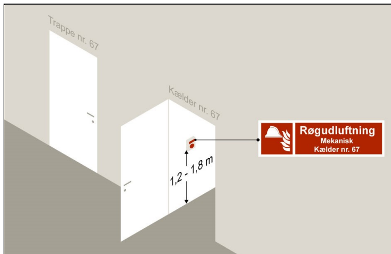
Figur 5.8.3.a: Eksempel på placering af aktiveringstryk til kælder
