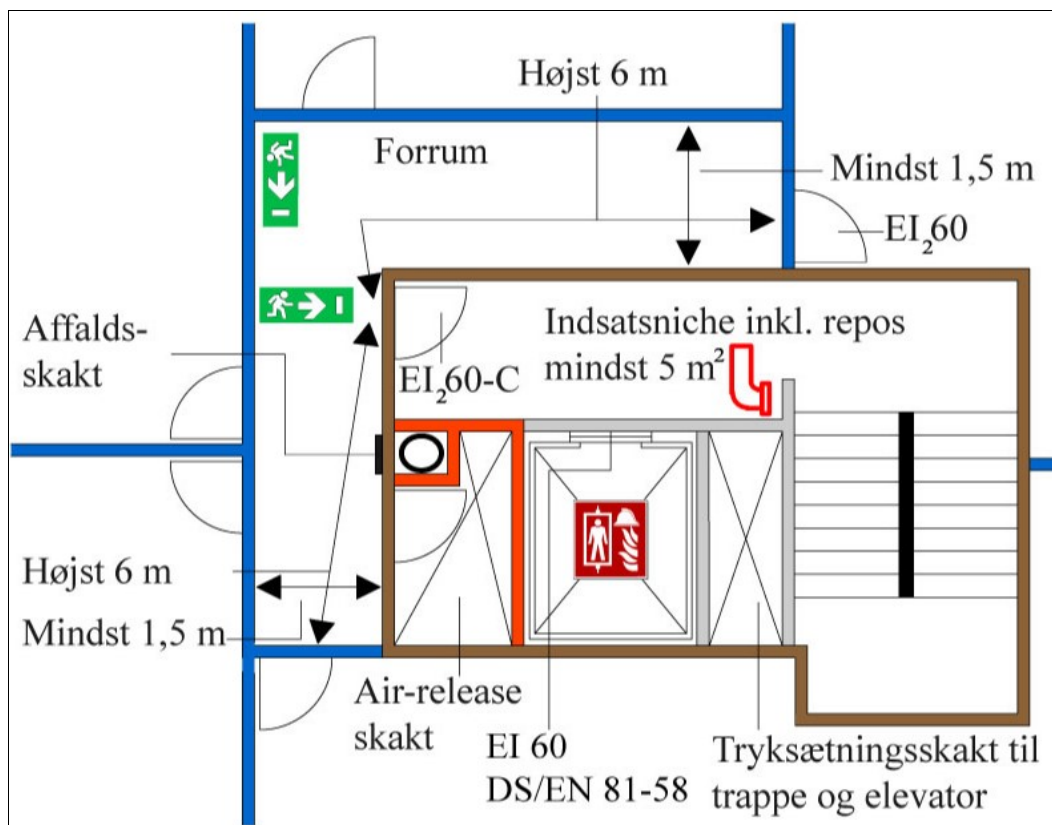
Figur 5.4.5.a: Eksempel på indretning af forrum med vinkel
