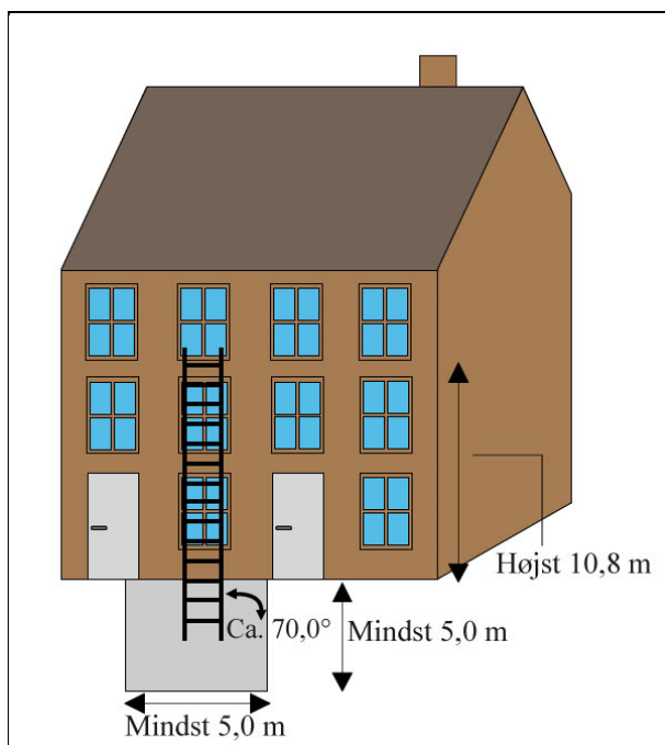
Figur 5.2.3.3.a: Opstilling af bærbar stige
