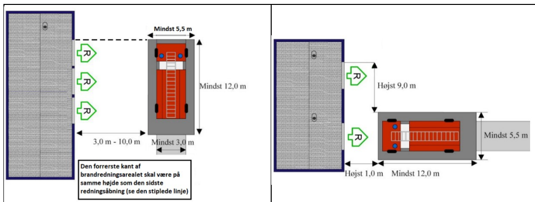
Figur 5.2.3.2.b: Afstand til bygning for kørbare stiger
